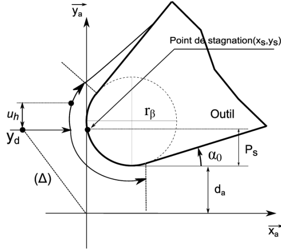
Figure 2-17. Trajectoire d'une particule de matière au-dessus et au-dessous du point de stagnation.
