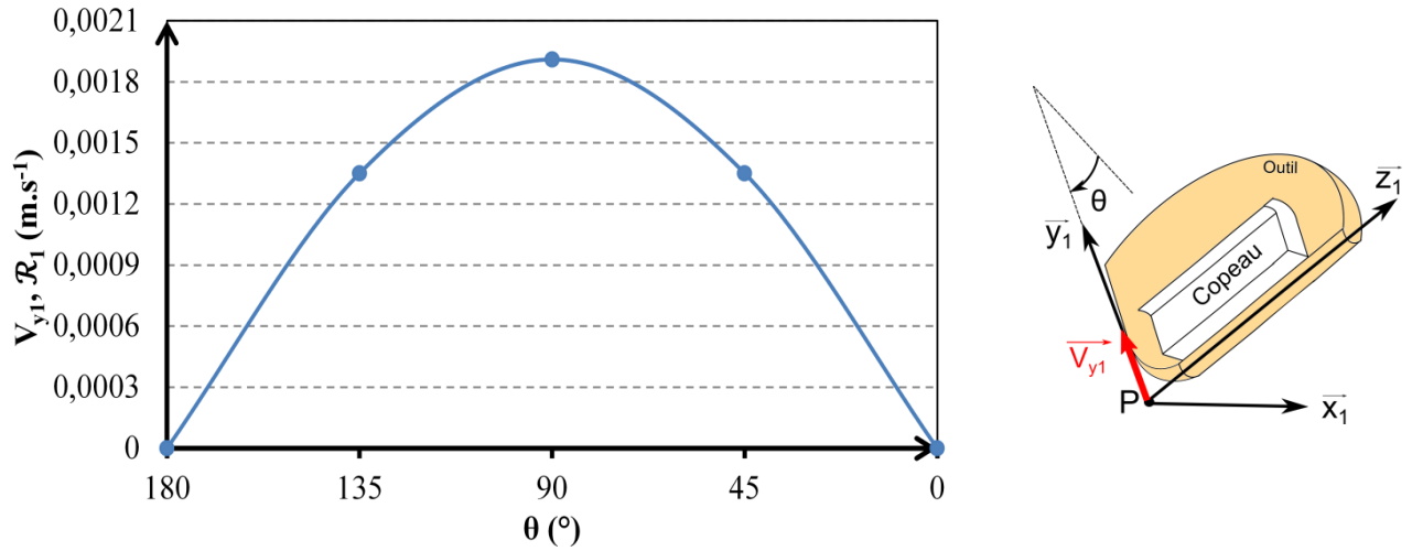
Figure 3-9. Variation de la composante normale à la plaquette portée par \bar{y}_1 au point P (pour les conditions de coupe du Tableau 3-3 et \kappa_r = 90^\circ, \gamma_0 = 0^\circ et \lambda_s = 0^\circ ).
