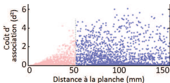
Figure 2.13 – Aperçu, sur un échantillon de traces d'abeilles (obtenues par le couple Filtre de Kalman + GNN), des coûts d'associations par rapport à la distance à la planche d'envol. Données issues de [Chiron 2013b].
