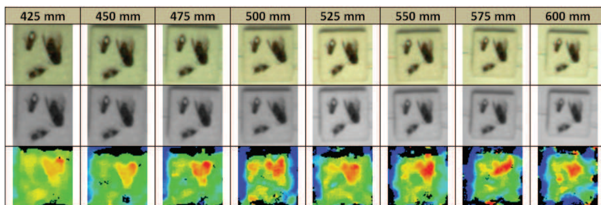
Figure D.2 – Spécimens vus par la caméra stéréo-vision TYZX G3 Evo placée à des distances bornées entre 42.5 cm et 60 cm. Première ligne : couleur, deuxième ligne : niveaux de gris, troisième ligne : carte de profondeur.
