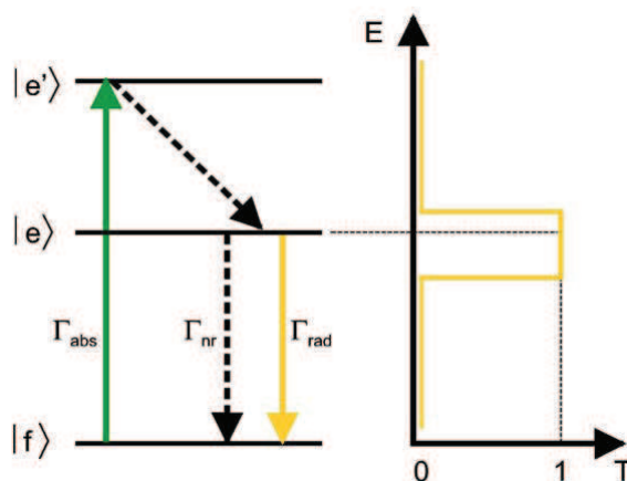
FIGURE 2.10 – Diagramme d'énergie schématisé d'un nano-objet individuel luminescent ; la courbe de transmission du filtre passe bande utilisé en microscopie de luminescence est représentée.
