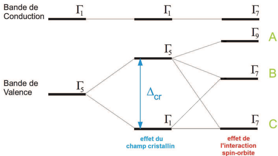
FIGURE 9.2 – Structure de bande d'un semi-conducteur blende de zinc au centre de la zone de Brillouin.
