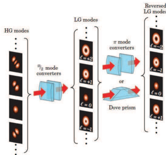
FIGURE 3.9 – Une paire de lentille cylindrique peuvent être utilisées pour convertir un mode de Hermite-Gauss (HG) en un mode de Laguerre-Gauss (LG). Comme la même paires de lentilles peut servir pour plusieurs modes de HG, une large gamme de mode de LG peut être créée. En augmentant la séparation entre les deux lentilles cylindriques on peut inverser le signe du moment orbital angulaire du mode de LG alors généré. Image extraite de [52].
