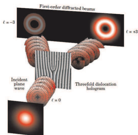
FIGURE 3.10 – Un hologramme peut produire un faisceau de front d'onde hélicoïdale possédant un moment orbital angulaire de charge l\hbar par photon. L'hologramme approprié peut être calculé, ou il peut être généré à partir du motif des interférences entre un faisceau possédant la forme spatiale désirée et une onde plane. Le motif d'holographie ainsi obtenu est comparable à un réseau de diffraction mais possède une dislocation de charge l sur l'axe optique (ici il y a une dislocation de 3). Lorsque l'hologramme est éclairé avec une onde plane, le premier ordre de diffraction possède le front d'onde hélicoïdal souhaité. Image extraite de [52].
