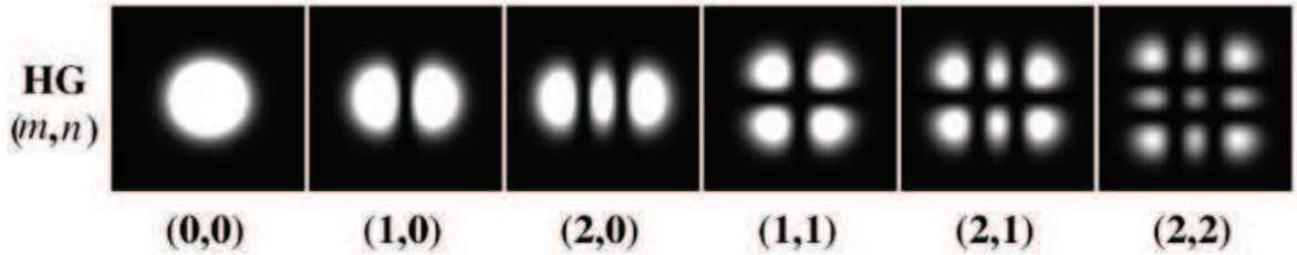
FIGURE 3.2 – Modes d'Hermite-Gauss décrits par leurs coefficients (m, n) .
