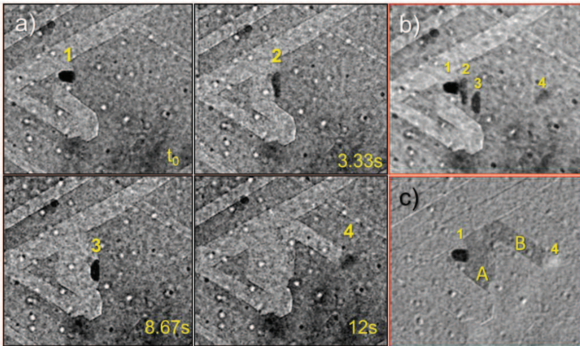
Figure 3.1. a) Série d'images consécutives à faible grossissement d'une nanoparticule qui enlève les atomes de carbone d'un bord de FLG parallèle avec celui-ci; b) Projection Z de la série d'images successives alignées du 3.1a ; c) Image calculée à l'aide de la première et de la dernière image dans 3.1a surlignant les régions de carbone qui ont réagi (zone A – récession des bords et zone B – découpe).
