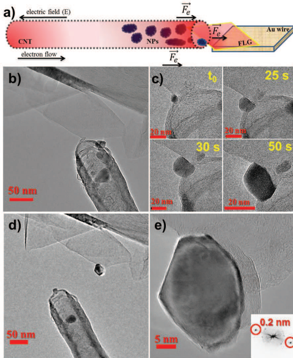
Figure 4.1. Dépôt contrôlé d'une nanoparticule métallique de Fe au bord d'une feuille de FLG. a) Représentation schématisée de l'expérience montrant les forces qui interviennent, une fois la différence de potentiel électrique appliquée. b) Le système CNT/FLG avant la déposition de la nanoparticule. c) Série d'images consécutives montrant la croissance de la nanoparticule au bord de la feuille de graphène (résolution temporelle 0,33s). d) Le système CNT/FLG après la déposition de la nanoparticule au bord du FLG. e) Image HR-TEM de la nanoparticule finale attachée au bord du FLG. L'analyse FFT (Fast Fourier Transform en anglais) permet de déduire un paramètre de réseau d'environ \sim 0.2 nm, caractéristique du Fe métallique dans les structures de type \phi et \gamma .
