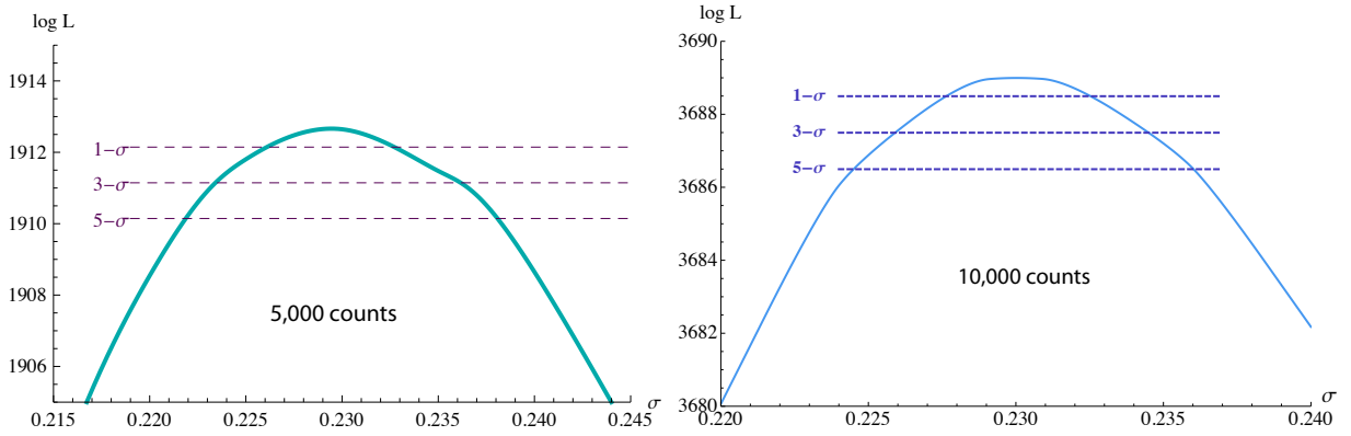
Figure B.12: Vraisemblance logarithmique d’une expérience comprenant 5000 (à gauche) ou 10 000 (à droite) sphères concentriques de rayon 10 et 11 Mpc/h mesurées dans notre simulation. Le modèle dépend ici seulement de la variance \sigma^2 ( \nu – qui paramétrise l’effondrement sphérique – et n – l’indice spectral – sont fixés). Les contours à 1,3 et 5 sigmas centrés sur la vraie valeur 0.23 sont représentés avec des tirets bleu foncé. Une expérience analogue mais en variant les trois paramètres pourrait être similairement envisagée.
