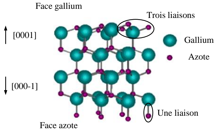
FIGURE 1.6 – Représentation schématique des deux polarités du nitride de gallium (extrait de [37]).
