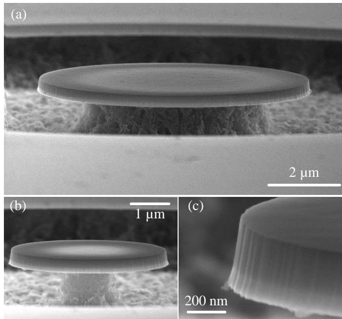
FIGURE 3.10 – Micrographie au microscope électronique au balayage d’un disque de 8\ \mu\text{m} de diamètre (a) et 3\ \mu\text{m} . (c) Zoom sur le bord du microdisque présenté en (b). Les images ont été réalisées par I. Roland à l’IEF.
