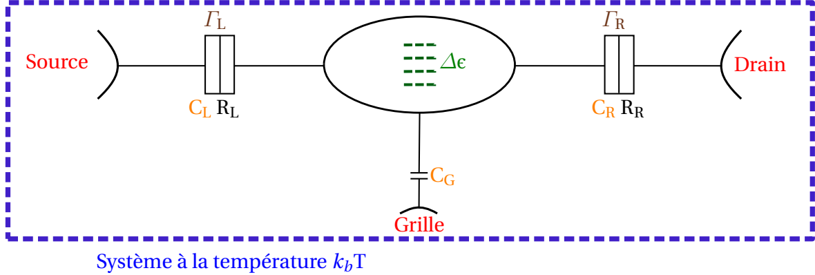
FIGURE 1.7 – Schéma électronique du nanotube de carbone en régime de boîte quantique avec les différentes électrodes. Les échelles d'énergie importantes rentrant en jeu sont mentionnées : la température k_bT , l'énergie de charge \frac{q^2}{C_\Sigma} , l'énergie des jonctions tunnel \Gamma et l'espacement de niveau dans la boîte \Delta\epsilon .
