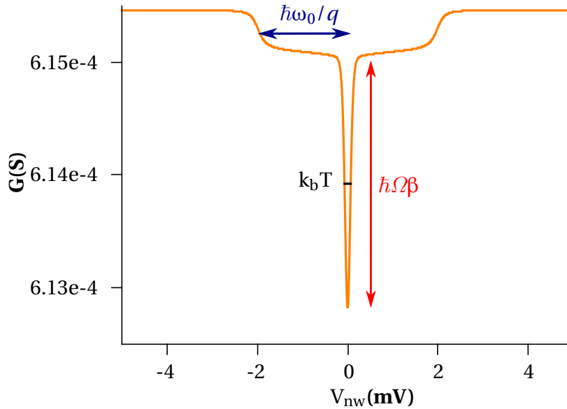
FIGURE E2 – Conductance G en fonction de la tension V_{nw} appliquée. L'intervention des échelles d'énergie du problème sont résumées sur le graphe, les interactions coulombiennes modélisées à travers \Omega modifient la profondeur du pic à énergie nulle, la température k_b T régule la largeur à mi hauteur du pic à énergie nulle et la fréquence de la cavité \hbar\omega_0 définit la longueur de la marche de conductance.
