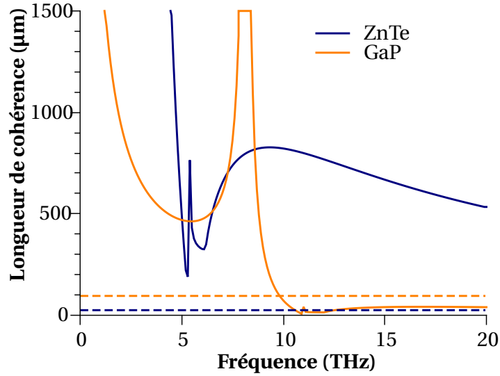
FIGURE 2.13 – Longueur de cohérence dans les cristaux de ZnTe en bleu et du GaP en orange. En pointillés ont été rajoutées les longueurs de cristaux utilisées pour le GaP de 100 \mu\text{m} (en orange) et le ZnTe de 20 \mu\text{m} (en bleu) pour la spectroscopie large bande.
