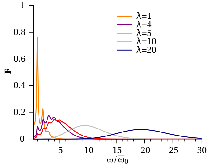
FIGURE 1.12 – Calcul de la fonction F modulante les taux de transition tunnel. Les paramètres utilisés sont Q = 5 et k_b T \rightarrow 0 . Les paramètres de couplage \lambda varient entre 0.5 et 20.
