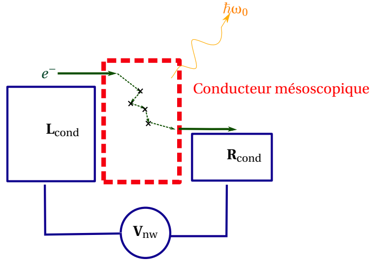
FIGURE F.1 – Représentation schématique d'un conducteur mésoscopique. L'électron se propage à travers les diffuseurs représentés par les croix noirs. Ces diffusions s'accompagnent de bruit qui entraînent des fluctuations de potentiel permettant l'émission de photons. La tension appliquée aux bornes de ce conducteur est V_{nw}
