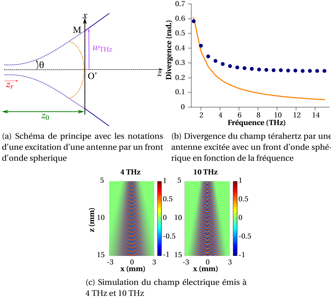
FIGURE 2.20 – Sur la figure (a), on définit le rayon du champ térahertz par w_{\text{THz}} ; en bleu continu nous avons le profil du champ en \frac{1}{e} qui est émis. Ce profil peut être relié à un champ virtuel gaussien en pointillé bleu de longueur de Rayleigh z_r et d'angle \theta et dont le centre de la zone de Rayleigh est situé à une distance z_0 de l'antenne (rayon minimal). Sur la figure (b) est représentée la divergence du champ térahertz calculée à partir de simulations numériques du champ émis par une antenne de 0.5 \mu\text{m} \times 0.5 \mu\text{m} excitée avec un faisceau infrarouge avec un front d'onde sphérique. Les points extraits de la simulations sont en bleus. En orange, nous avons tracé la loi \tan \psi \sim \psi = \sqrt{2} \left( \frac{\sqrt{2}c}{\pi f_{\text{THz}} w_{\text{opt}}} \right) , où w_{\text{opt}} = 0.25 \mu\text{m} que suit la divergence si l'antenne est excitée par un faisceau faiblement divergent. A noter que le passage de \theta à \psi s'effectue en multipliant par \sqrt{2} . A la figure (c) sont présentés les calculs des champs émis à 4 THz et 10 THz en champ lointain.
