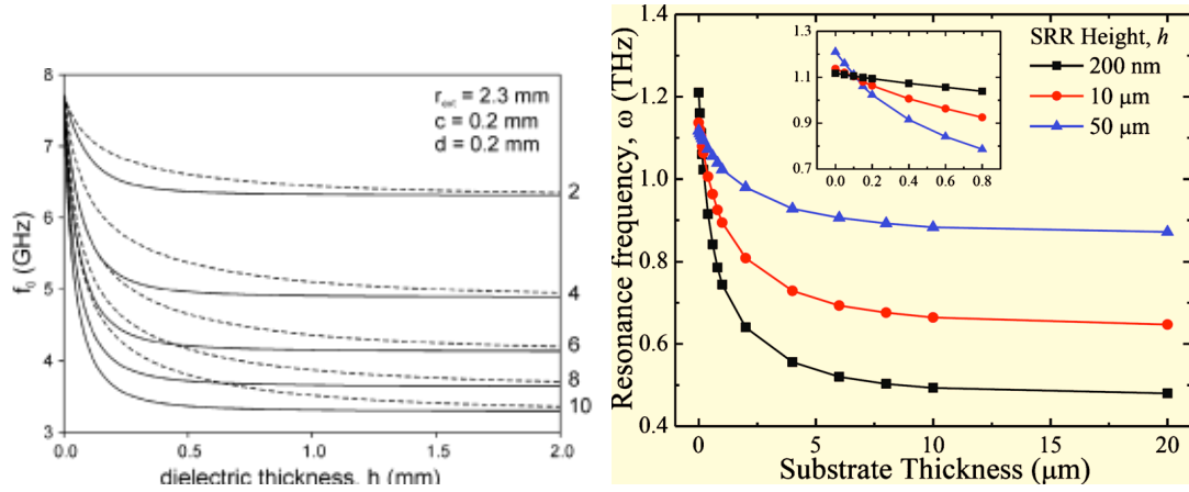
(a) Figure 6 (a) extraite de l'article de Baeana et al. [125] montrant la dépendance de la fréquence de résonance LC en fonction de l'épaisseur du substrat et différentes valeurs de permittivité diélectrique indiquées à droite.
