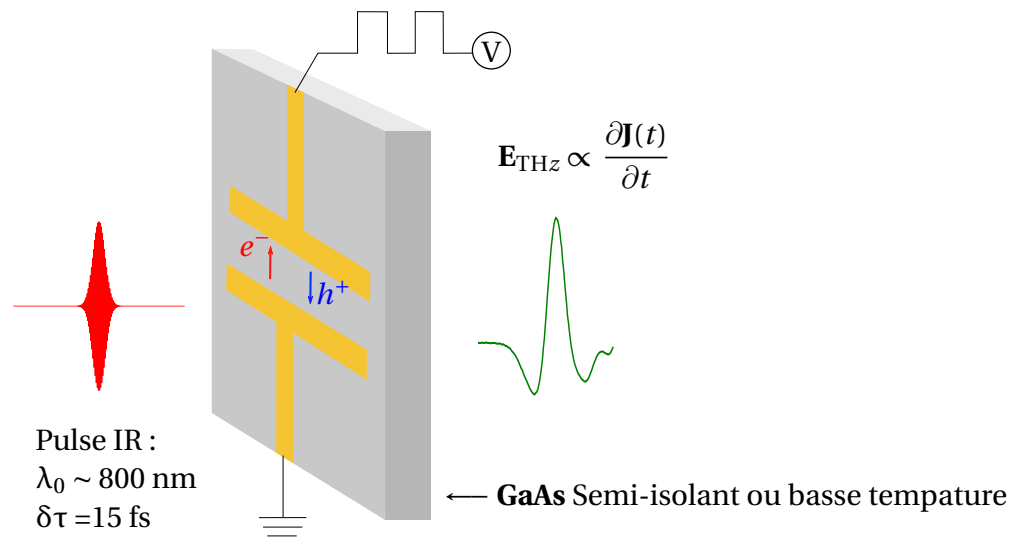
FIGURE 2.9 – Schéma d'une antenne photoconductrice dipolaire sur du GaAs semi-isolant (SI) ou basse température (BT) excitée par une impulsion infrarouge femtoseconde. Le faisceau infrarouge génère des porteurs qui sont accélérés par le champ électrique aux bornes de l'antenne.
