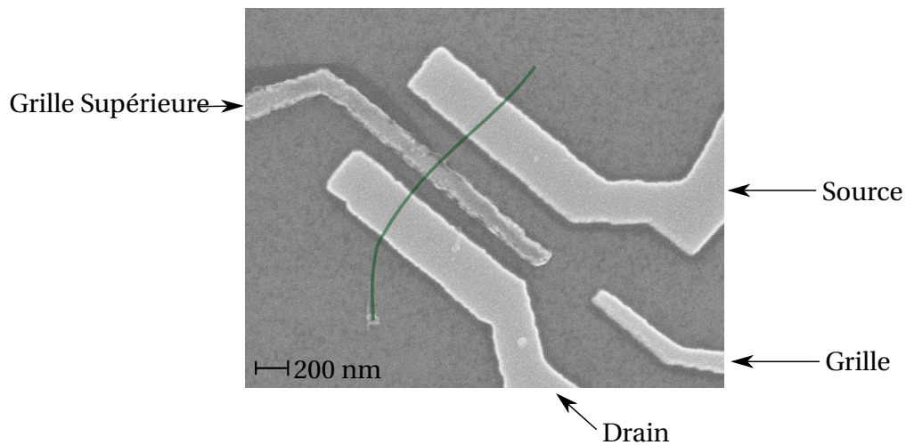
FIGURE C.2 – Photographie prise au microscope électronique à balayage du nanotube de carbone contacté par les électrodes de source et drain avec la grille supérieure et la grille. La nanotube signalé en vert afin de mieux visualiser sa position sur l'échantillon.
