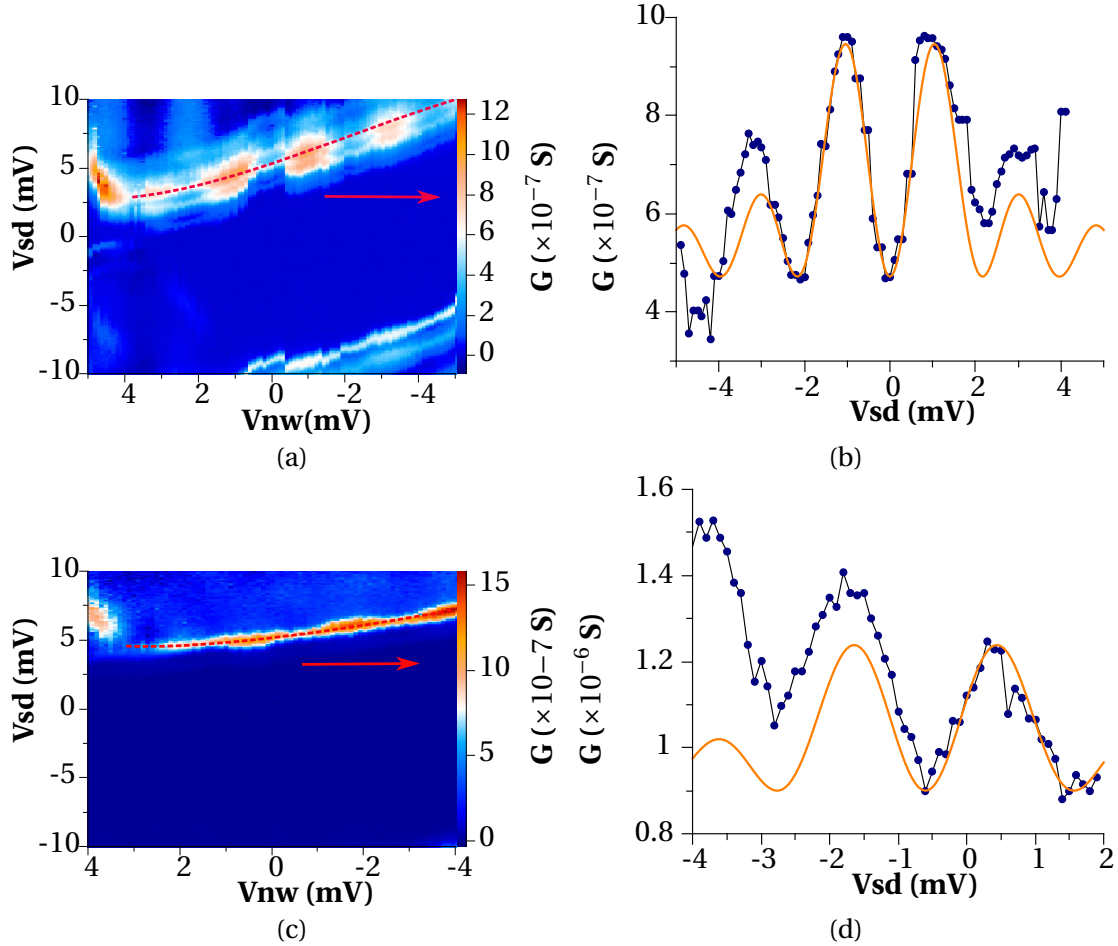
FIGURE 4.8 – Etude de l'évolution des niveaux électroniques en fonction de V_{nw} . En (a), nous avons un diagramme de stabilité pris à V_g = 1.19 V en faisant varier V_{sd} \in [-10 \text{ mV}, 10 \text{ mV}] et V_{nw} \in [-5 \text{ mV}, 5 \text{ mV}] . La figure à sa gauche est une coupe du niveau électronique dessinée en pointillée rouge. Nous avons rajouter dessus une fonction de Bessel d'ordre 1 en orange. En (b), nous avons un second diagramme de stabilité pris à V_g = 1.21 V en faisant varier V_{sd} \in [-10 \text{ mV}, 10 \text{ mV}] et V_{nw} \in [-5 \text{ mV}, 5 \text{ mV}] . La figure à sa gauche est une coupe du niveau électronique dessinée en pointillées rouges sur laquelle nous avons rajouter une fonction de Bessel d'ordre 1 en orange.
