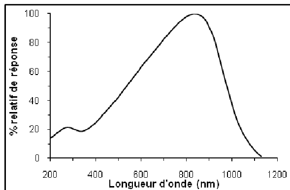
Figure II-7 : réponse spectrale de la photodiode Newport, modèle 818-BB-22 (données constructeur).
