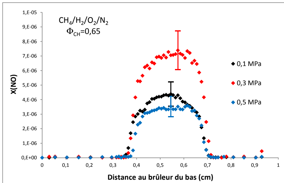
Figure IV-28 : Profils de fraction molaire de NO mesurés dans la flamme \text{CH}_4/\text{H}_2/\text{air} riche ( \Phi_{\text{CH}} = 0,65 ) en fonction de la pression (de 0,1 à 0,5 MPa).
