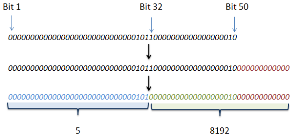
Figure IV.7 – Conversion d’un fingerprint binaire vers une représentation sous forme de liste d’entiers permettant un stockage plus compact dans la base de données. On fait l’hypothèse ici qu’un fingerprint de 50 bits doit être inséré dans la base. Il est nécessaire d’ajouter des bits à 0 (en rouge) pour ce fingerprint afin de le représenter sous la forme de deux entiers 32 bits. On obtient ainsi deux entiers qui peuvent être aisément stockés en base de données.
