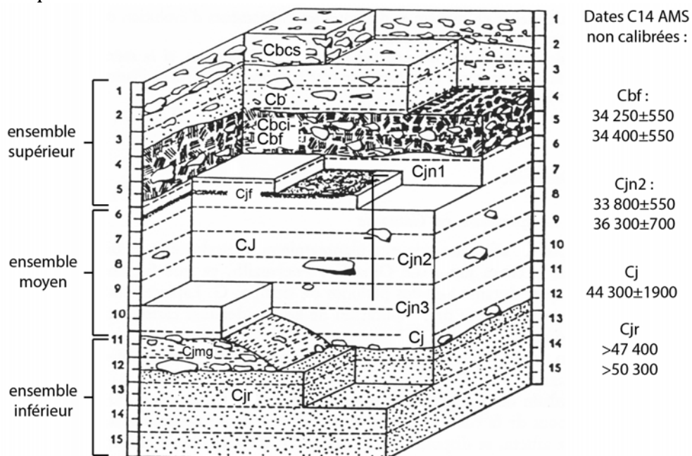
Fig. 290 : Stratigraphie théorique de la grotte de Gatzarria (d'après Laplace, 1971). Datations d'après Barshay-Szmidt et al. 2012, sauf Cj, d'après Ready, 2013.
