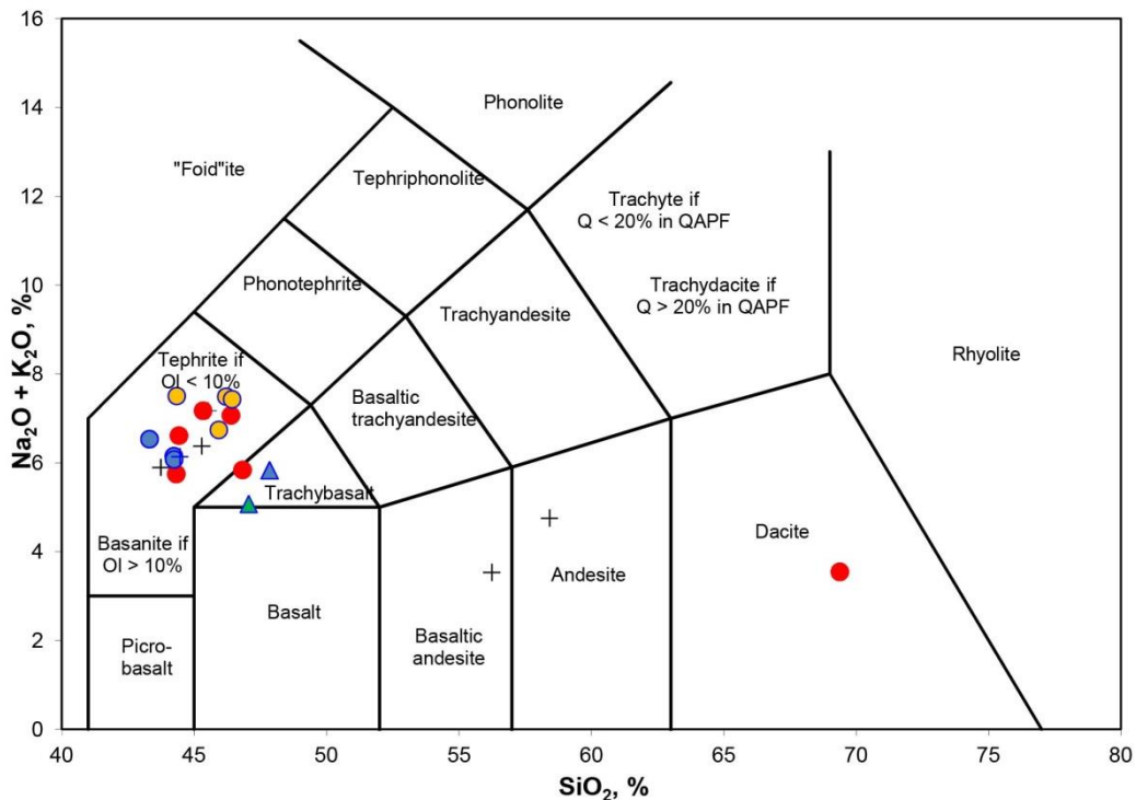
Figure V.3 : Diagramme somme des alcalins versus SiO 2 (TAS), d'après Le Bas et al. (1986) pour les laves d'Ardèche. Les croix correspondent aux échantillons datés uniquement en K-Ar, les cercles aux échantillons datés en K-Ar et ^{40}\text{Ar}/^{39}\text{Ar} . En bleu sont reportés les échantillons pas contaminés (voir texte), en orange les échantillons modérément contaminés, en rouge les échantillons les plus contaminés.
