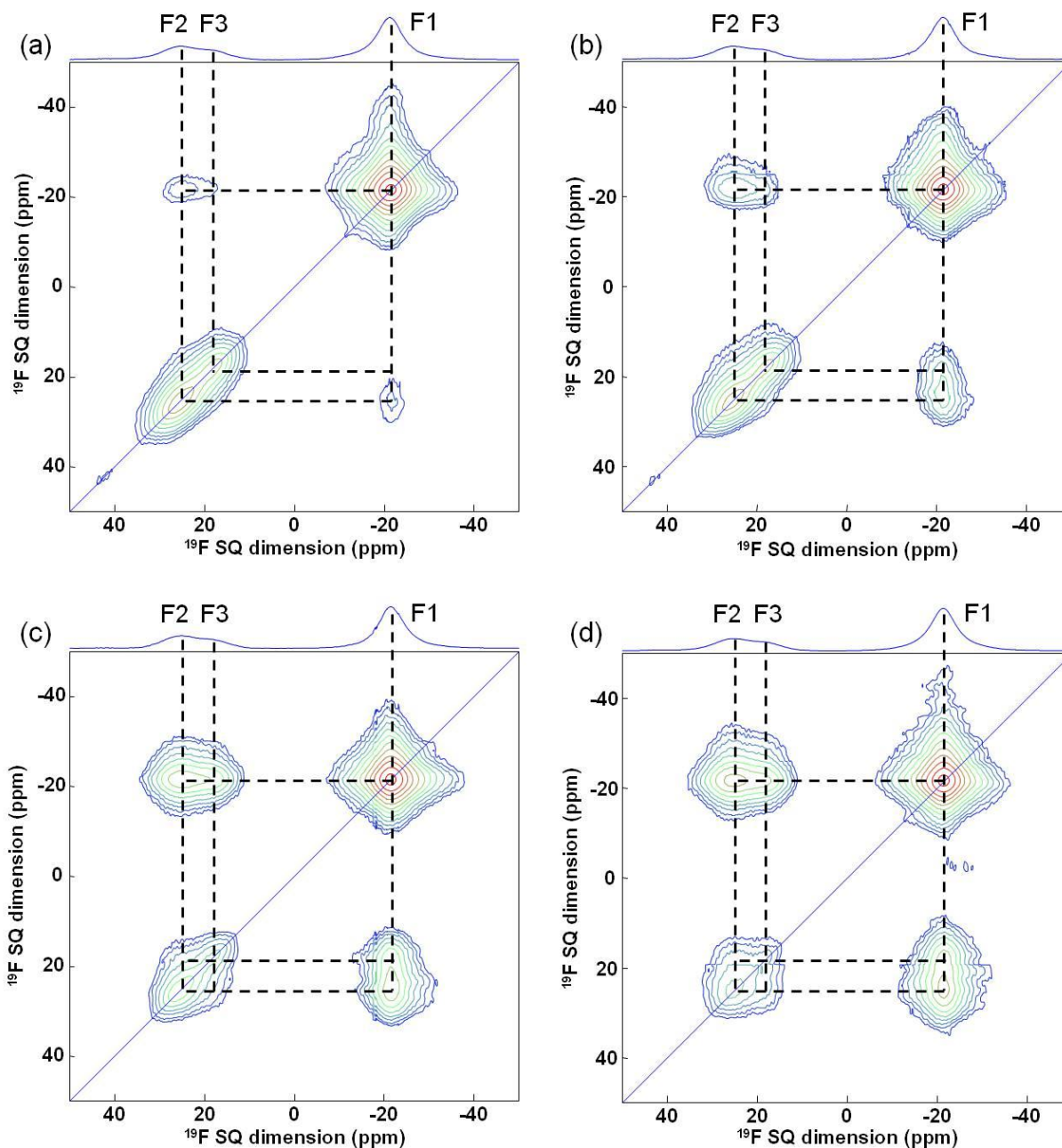
Figure 15 : Spectres 2D EXSY MAS (44 kHz) de ^{19}\text{F} de \text{La}_{0.97}\text{Ba}_{0.03}\text{F}_{2.97} , enregistrés à 40^\circ\text{C} et pour des temps de mélanges de (a) 250\ \mu\text{s} , (b) 500\ \mu\text{s} , (c) 2\ \text{ms} et (d) 5\ \text{ms} . Leur projection complète sur l'axe ^{19}\text{F} MAS 1D est représentée au-dessus d'eux. Les droites continues situent la diagonale ; celles en tiret marquent les pics hors diagonale (matérialisant les échanges).
