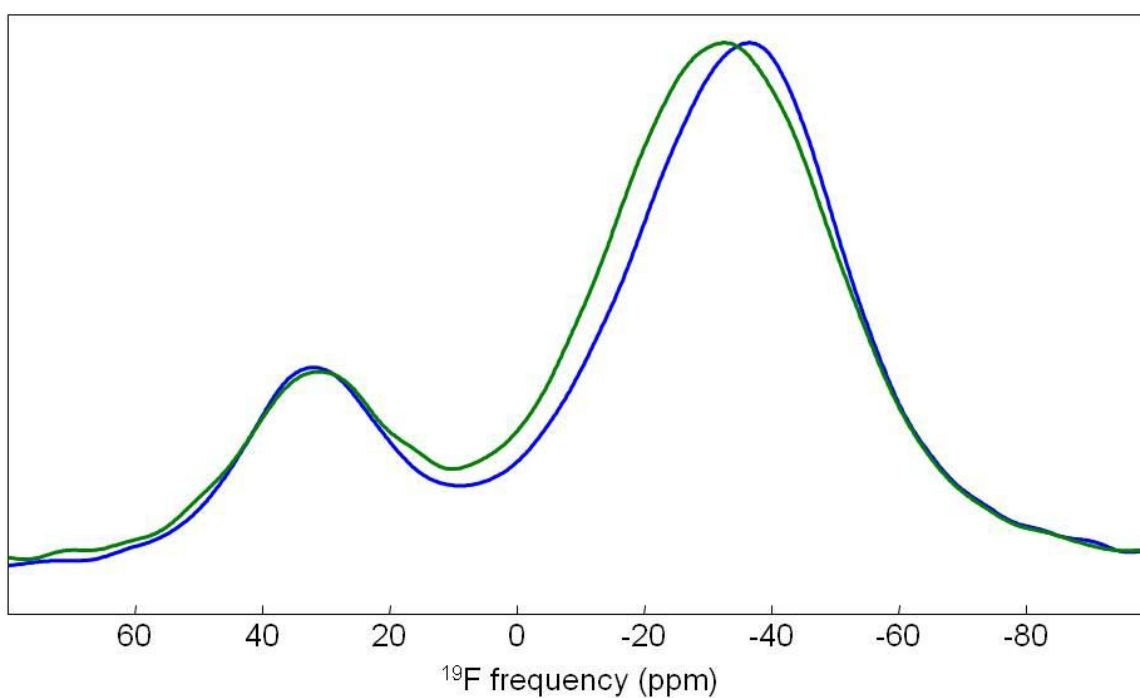
Figure 31 : Spectres RMN ^{19}\text{F} MAS de \text{CeF}_3 à 64°C (64 kHz, en bleu) et 51°C (54 kHz, en vert).
