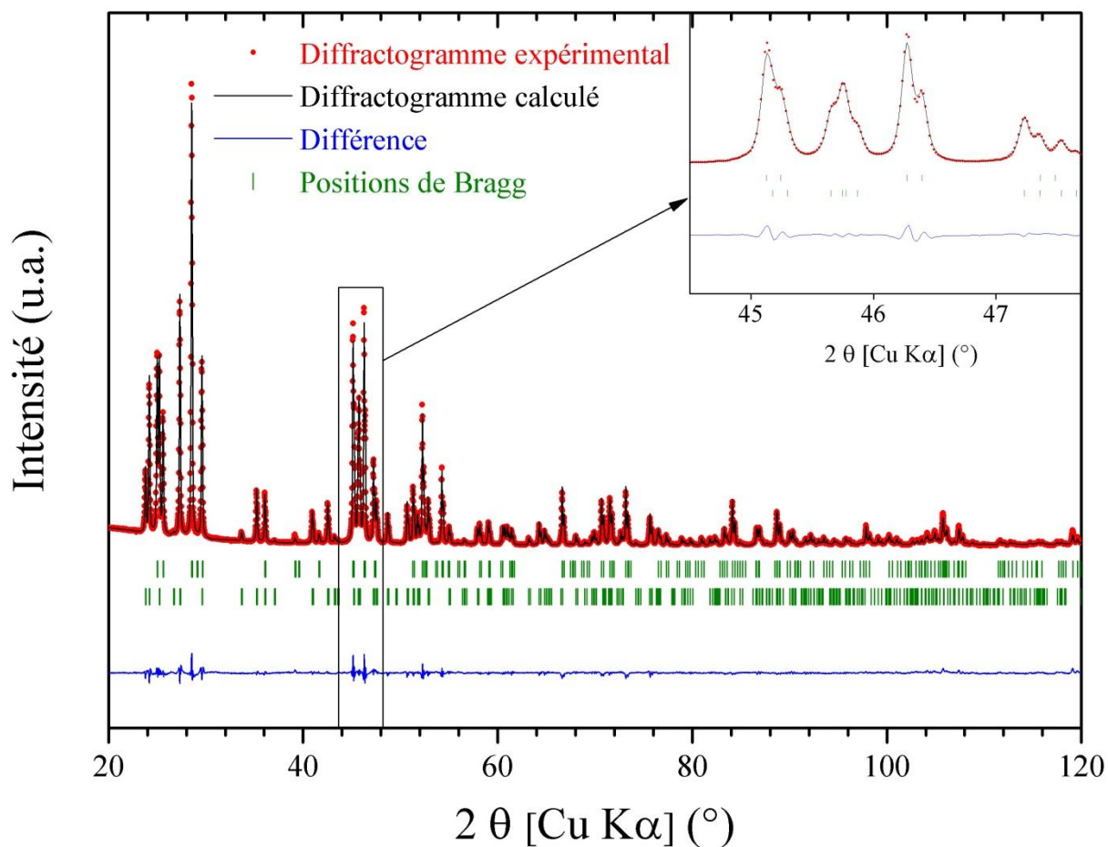
Figure 28 : Diffraction RX (expérimental et calculé) du mélange \text{SmF}_3 , de structure tysonite (49% en masse) et orthorhombique (51% en masse).
