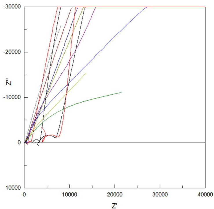
Figure 46 : Capture d'écran de la représentation de l'impédance d'une pastille frittée de \text{Ce}_{0.95}\text{Sr}_{0.05}\text{F}_{2.95} mécanosynthétisé dans un diagramme de Nyquist lors d'une mesure d'impédance (cf. programme en Figure 10 ).
