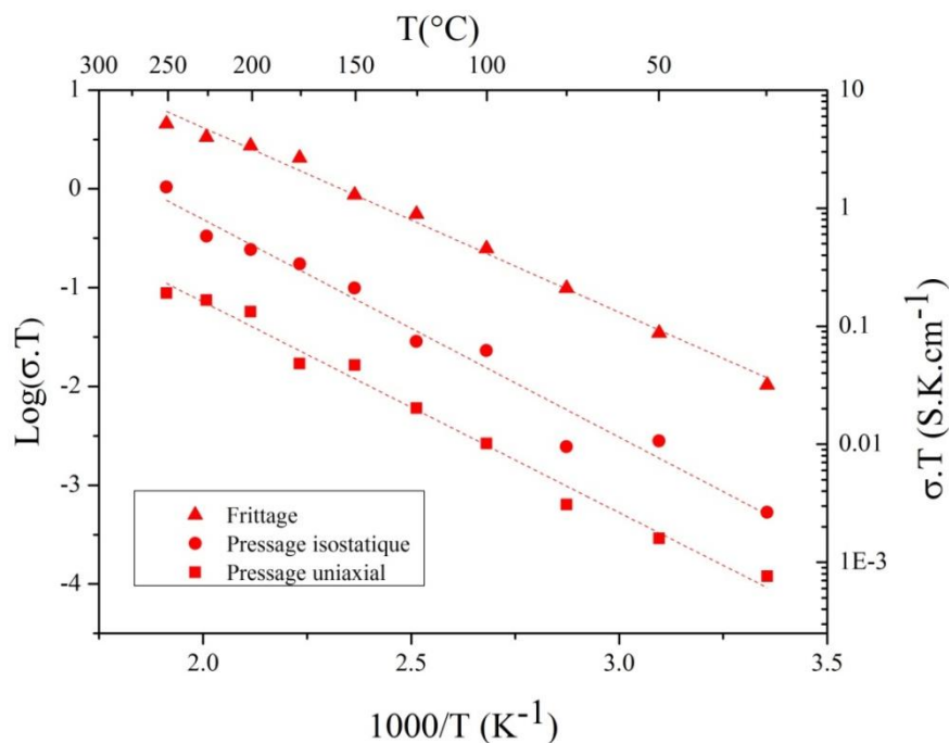
Figure 24 : Diagramme d'Arrhenius de la conductivité ionique du composé La_{0,95}Ba_{0,05}F_{2,95} obtenu pour des échantillons microcristallins suivant trois techniques de mise en forme.
