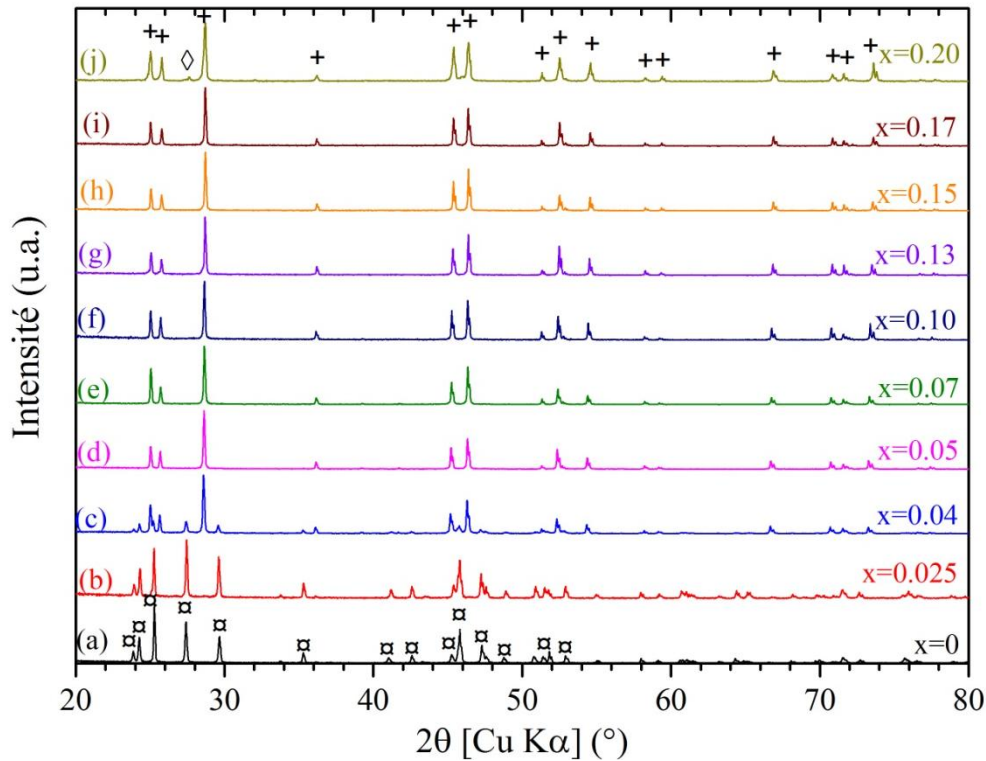
Figure 1 : Diagrammes DRX des composés de la solution solide Sm_{1-x}Ca_xF_{3-x} ( 0 \leq x \leq 0.20 ) obtenus par synthèse à l'état solide ( 1000^\circ C , 24 h suivie d'une trempe, excepté pour SmF_3 ). Les trois phases identifiées sont représentées par les symboles suivants : + pour la phase de type tysonite, \square pour la phase de type orthorhombique et \diamond pour la phase de type fluorine Ca_{1-y}Sm_yF_{2+y} .
