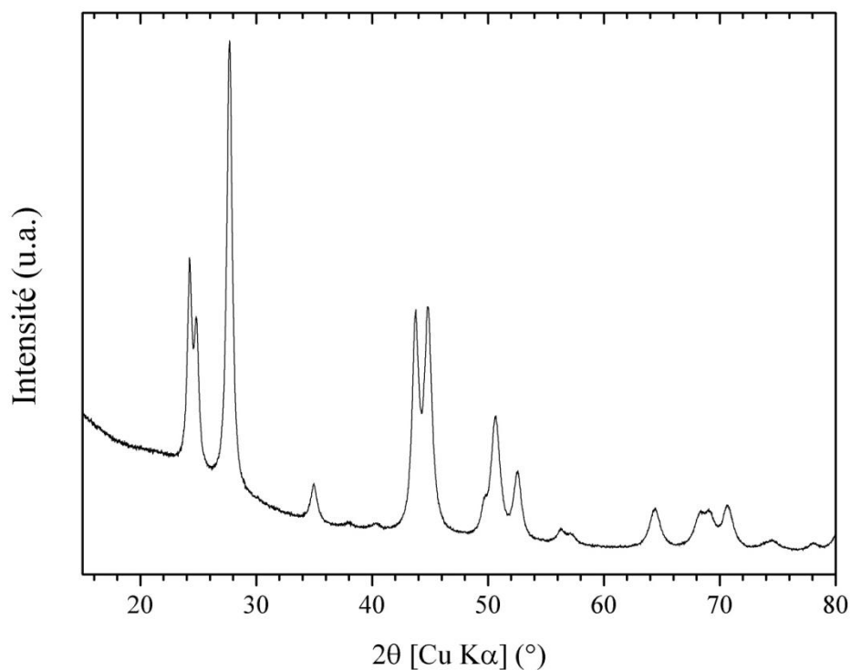
Figure 38 : Diffractionogramme DRX de \text{La}_{0.95}\text{Ca}_{0.05}\text{F}_{2.95} nanosynthétisé par broyage (12 h, 400 rpm, en milieu sec, dans une jarre en zircone, sous 10 billes).
