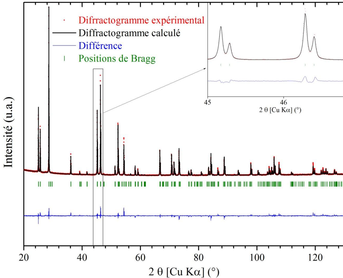
Figure 7 : Diffraction DRX (expérimental et calculé) de Sm 0.95 Ca 0.05 F 2.95 .
