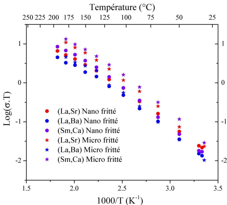
Figure 39 : Diagrammes d'Arrhenius de la conductivité ionique des solutions solides de type tysonite RE_{1-x}M_xF_{3-x} ( RE = La, Sm, Ce ; M = Ba, Ca, Sr ) pour x = 0.05 , pour des échantillons nanosynthétisés frittés (étoiles) et microcristallins frittés (ronds).
