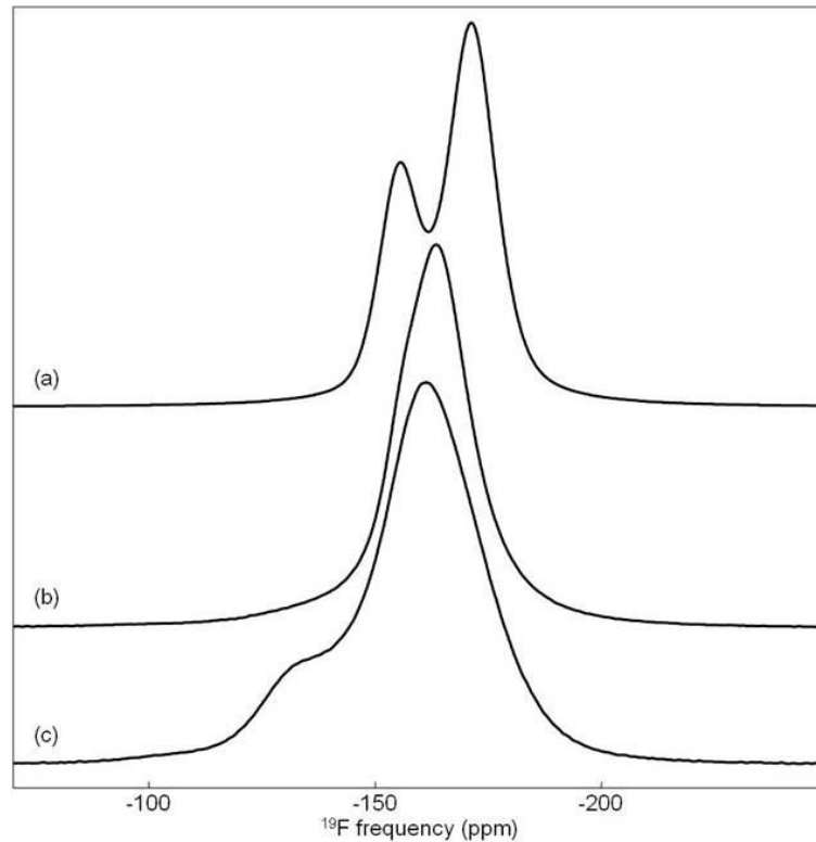
Figure 20 : Spectres RMN MAS (64 kHz, 64°C) de 19 F de (a) SmF 3 de structure tysonite (spectre déduit de la reconstruction de celui du mélange SmF 3 orthorhombique-tysonite), (b) Sm 0.95 Ca 0.05 F 2.95 et (c) Sm 0.85 Ca 0.15 F 2.85 . Les spectres sont normés par rapport au pic le plus intense.
