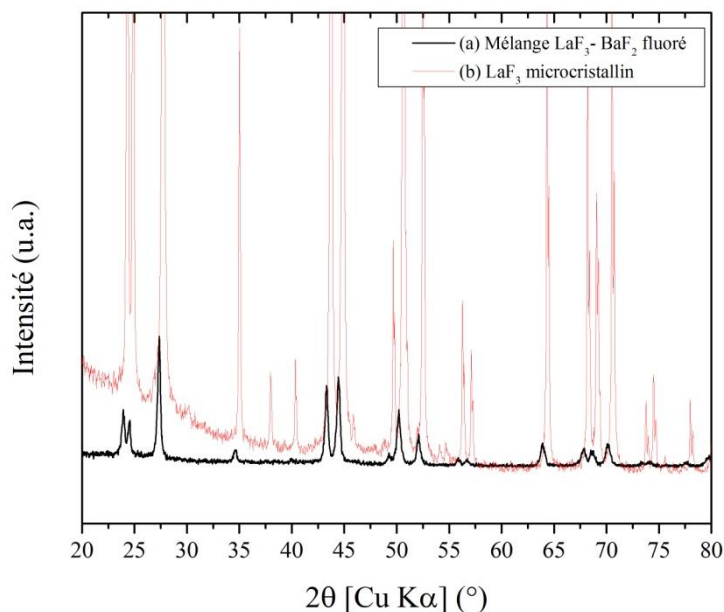
Figure 29 : Diagramme DRX (noir) d'un mélange LaF_3 + BaF_2 synthétisé à partir de précurseurs acétates ( Tableau 14 ) et fluoré à 500^\circ C pendant 5h sous 50% de F_2 , par rapport à la référence LaF_3 (diagramme rouge).
