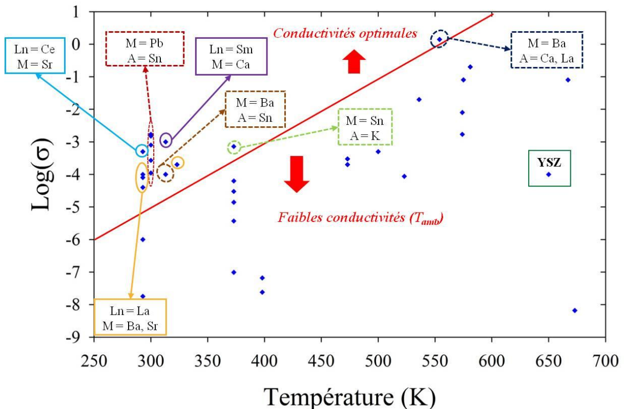
Figure 6 : Relevé des valeurs de conductivité ionique en fonction de la température des meilleurs électrolytes fluorés (19-30) (structures fluorine \text{M}_{1-x}\text{A}_x\text{F}_{2+x} : traits pointillés ; structure tysonite \text{Ln}_{1-x}\text{M}_x\text{F}_{3-x} : traits pleins). Pour comparaison, la référence oxyde YSZ est donnée (cadre vert foncé). La droite rouge est une limite arbitraire fixée pour identifier les électrolytes jugés les plus pertinents dans le cadre de notre projet (cf. IV.3 ). Pour plus de détails, voir le tableau de valeurs en Annexes .
