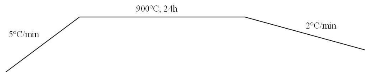
Figure 3 : Représentation du programme usuel de chauffage des tubes de platine
