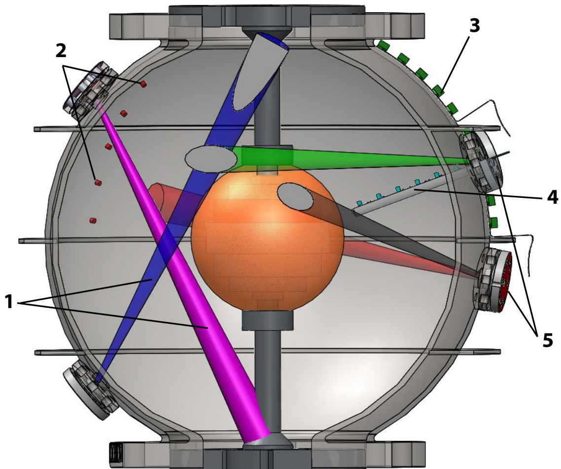
FIGURE 2.2 – Vue 3D des deux sphères de l'expérience DTS ainsi que l'ensemble de l'appareillage de mesure. On peut trouver (1). Des mesures directes de la vitesse du fluide par des tirs Doppler ultrason. Ils sont représentés en couleur le long de leur trajet dans le volume fluide. (2). On peut mesurer le potentiel électrique à la surface de la sphère externe en 5 points de latitude. (3). Magnétomètres GMR (magnétorésistance géante) permettant de mesurer les trois composantes du champ magnétique. (4). Doigt de gant et ses 10 capteurs magnétiques à effet Hall. (5). Bouchons étanches pouvant accueillir indifféremment des sondes Doppler ultrasonores ou le doigt de gant.
