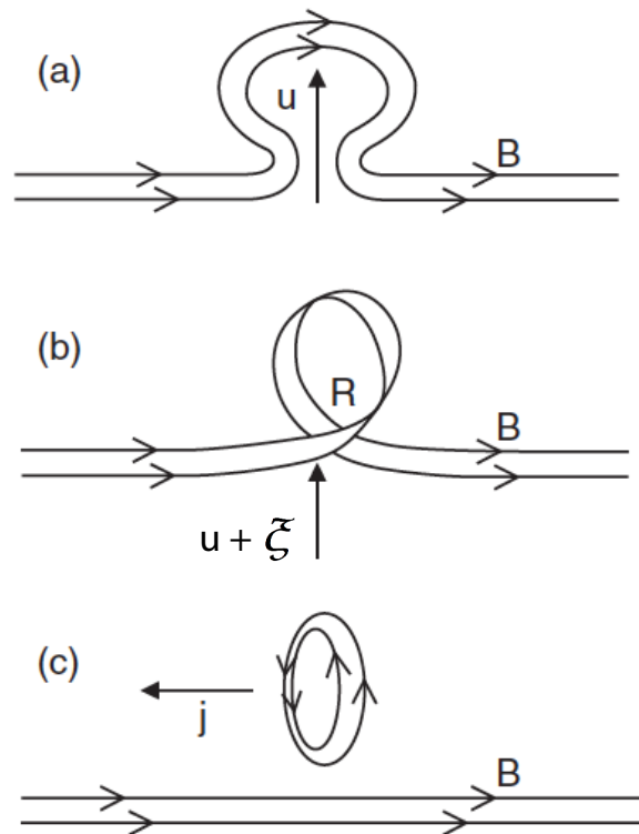
FIGURE 6.1 – Mécanisme d'induction de Parker combinant l'action couplée d'un champ vitesse u et de sa vorticité \zeta . Ce mécanisme représente le mécanisme d'induction \alpha discuté dans le texte. Schéma Roberts et King (2013)
