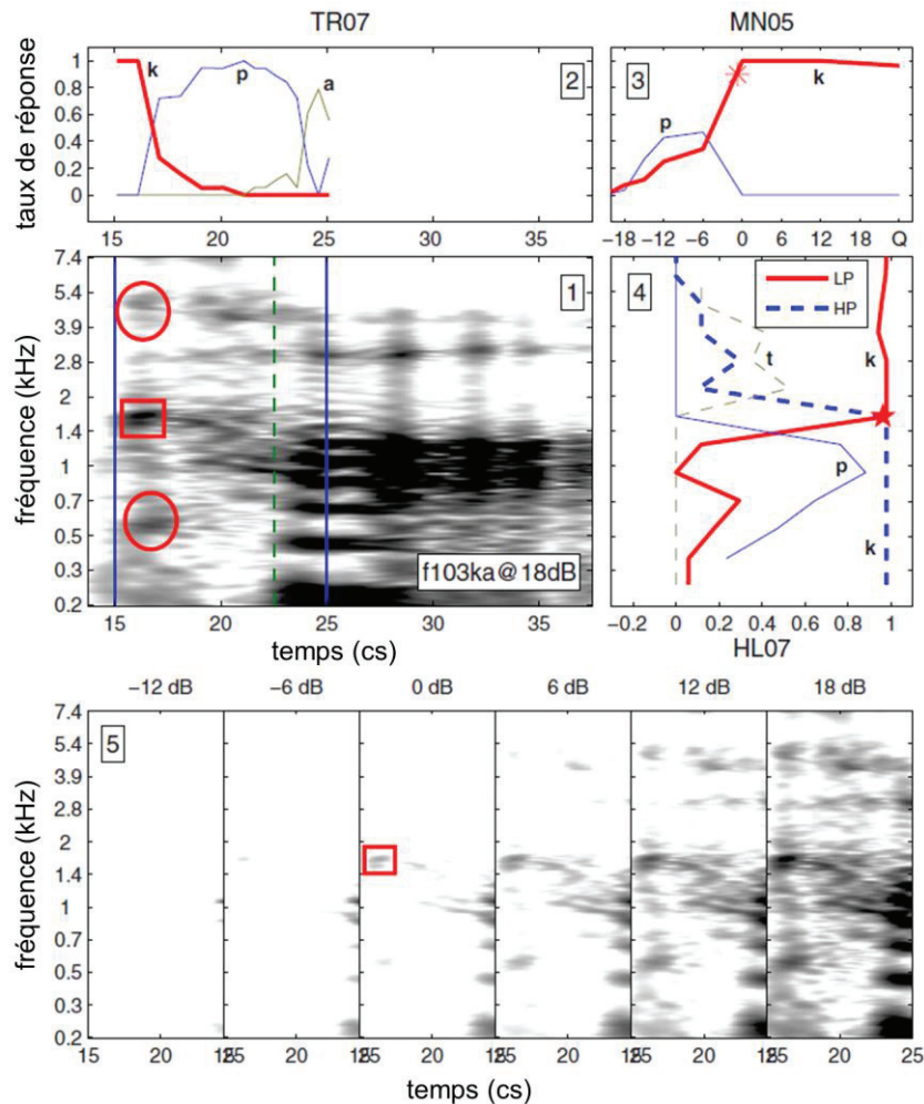
Figure 18 – Résultat de l’analyse 3DDS pour une production de la syllabe /ka/. Adapté de (Li et al., 2010). (1) représentation temps-fréquence du stimulus (AI-gram à 18 dB SNR). L’indice acoustique identifié est encadré en rouge et les indices conflictuels sont marqués par des ellipses. Le trait vert indique approximativement le début de la voyelle et les traits bleus la plage considérée pour les troncatures. (2) Profil de confusion obtenu lors de la troncature progressive du segment initial (taux de réponses correctes en rouge). (3) Profil de confusion obtenu lors du masquage progressif du stimulus (taux de réponses correctes en rouge). (4) Profils de confusion obtenus lors du filtrage progressif passe-bas (traits continus, taux de réponses correctes en rouge) ou passe-haut (traits discontinus, taux de réponses correctes en bleu) du stimulus. (5) Représentation du stimulus à différents SNRs (AI-grams).
