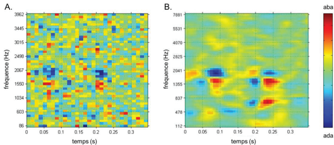
Figure 25 – ACIs correspondant à la catégorisation /aba/-/ada/, pour le participant LV de l'étude 1. A. ACI dérivée en utilisant l'algorithme de l'étude 1 (calcul basé sur le spectrogramme des bruits, 2 hyperparamètres). B. ACI dérivée en utilisant l'algorithme de l'étude 4 (calcul basé sur le cochléogramme des stimuli, 1 seul hyperparamètre).
