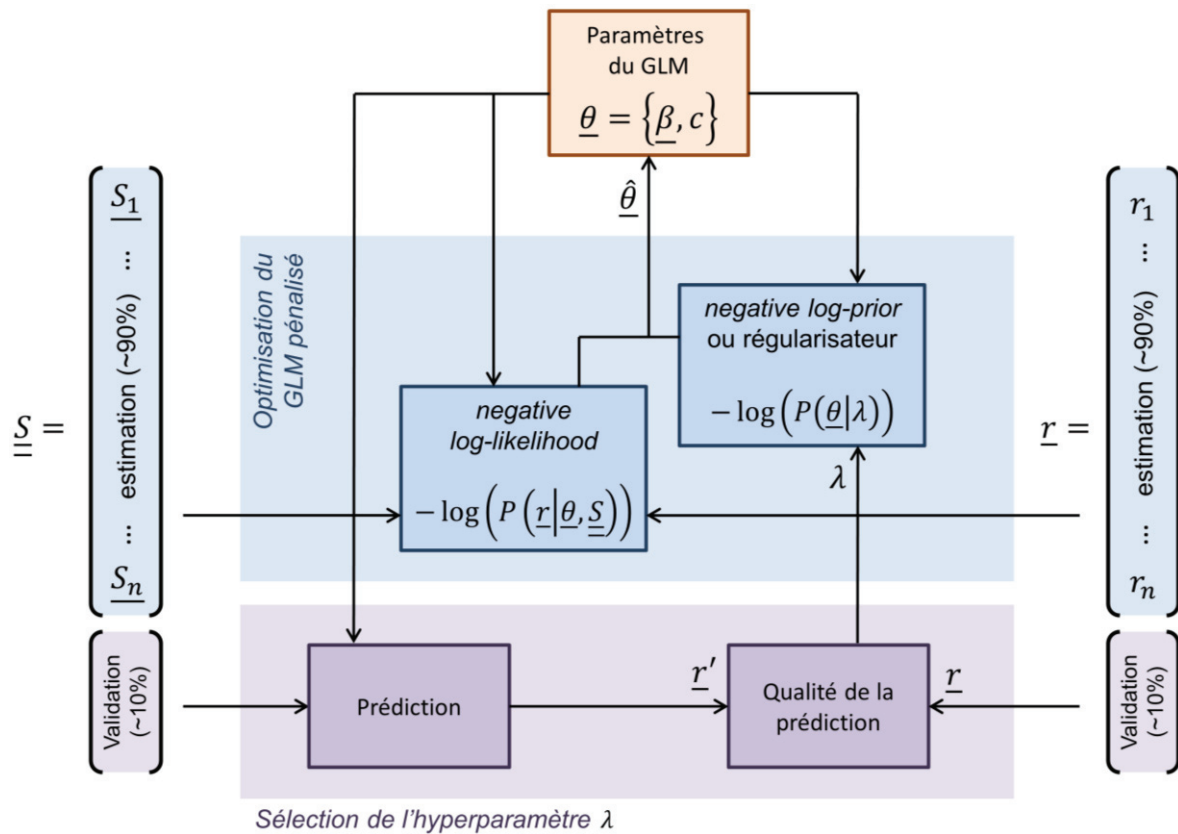
Figure 24 - Représentation schématique de la procédure de l'estimation de CI visuelles par GLM pénalisé.
