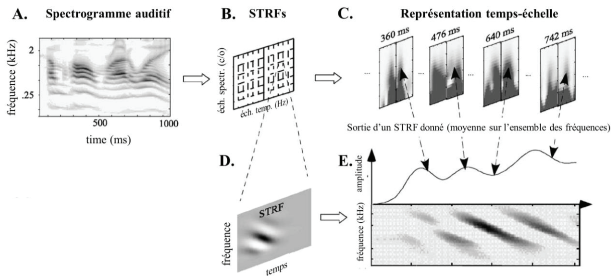
Figure 15 – Représentation schématique du calcul de la représentation multi-résolution pour la phrase « Come home right away ». A. Spectrogramme auditif du stimulus. B. Banque de filtres STRFs. C. Représentation corticale (temps-échelle). Chaque tranche correspond à une visualisation, à un instant donné, du signal dans l'espace échelle temporelle – échelle spectrale. D. Exemple d'un filtre STRF particulier (pour une valeur donnée de modulation temporelle et de modulation spectrale). E. Activation au cours du temps de ce filtre STRF, positionné à différentes fréquences, suite à la présentation du stimulus. Adapté de (Elhilali et al., 2003)
