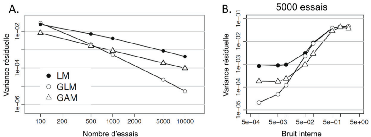
Figure 22 - Effets du nombre d'essais et du bruit interne sur la qualité de l'estimation, exprimée en variance résiduelle (distance entre la CI et le gabarit réel), pour un observateur linéaire simulé. Trois méthodes sont représentées : la corrélation inversée (cercle noir), le GLM (cercle blanc), et le GLM pénalisé ou GAM (triangle blanc). A. Évolution de la variance résiduelle en fonction du nombre d'essais pour un observateur linéaire sans bruit interne. B. Évolution de la variance résiduelle en fonction du bruit interne pour une passation de 5000 essais. Adapté de (Knoblauch & Maloney, 2012).
