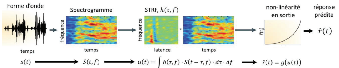
Figure 19 - Diagramme du modèle de neurone auditif basé sur le STRF, sans filtre post-décharge. Les étapes du traitement correspondent au calcul du spectrogramme S(t, f) à partir de la forme d'onde, la convolution avec le STRF h(\tau, f) , puis la prédiction de la probabilité de décharge \hat{r}(t) par une transformation non linéaire du résultat. Adapté de (Theunissen & Elie, 2014).
