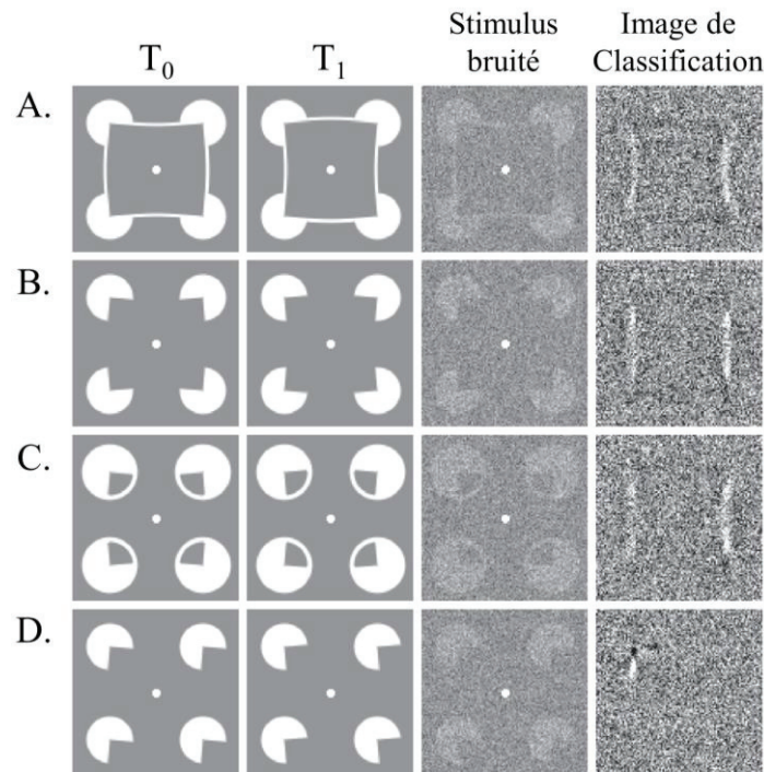
Figure 20 - Couples de cibles T0 et T1 utilisés dans l'expérience de perception des contours illusoires (Gold et al., 2000), pour les différentes conditions. Dans chaque cas, un exemple de stimuli et l'Image de Classification obtenue. A. Contours complets. B-C. Contours illusoires (contour de Kanizsa et contour de Kanizsa masqué). D. Stimulus fragmenté, sans contour illusoire. Adapté de (Murray et al., 2005).
