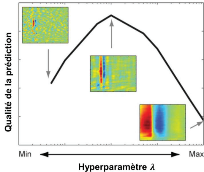
Figure 23 – Exemple de calcul d’un STRF par Régression Pénalisée. Qualité de la prédiction en fonction de la valeur de l’hyperparamètre \lambda . Les estimations correspondant à trois valeurs de \lambda sont représentées. Adapté de (Wu et al., 2006).
