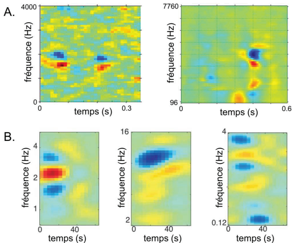
Figure 27 – Rapprochement entre les ACIs et les STRFs. A. Exemples d’ACIs issues des études précédentes (gauche : tâche de catégorisation /aba/-/ada/ ; droite : tâche de catégorisation /da-/ga/ en contexte /al/ et /aʁ/). B. Exemples de STRFs de neurones auditifs du cortex auditif primaire obtenus pour des tâches d’écoute passives chez le furet, adaptés de (Fritz et al., 2003). L’échelle couleur représente la probabilité de réponse dans A. et la probabilité de décharge dans B. Tous les axes fréquentiels sont logarithmiques excepté celui de la première ACI.
