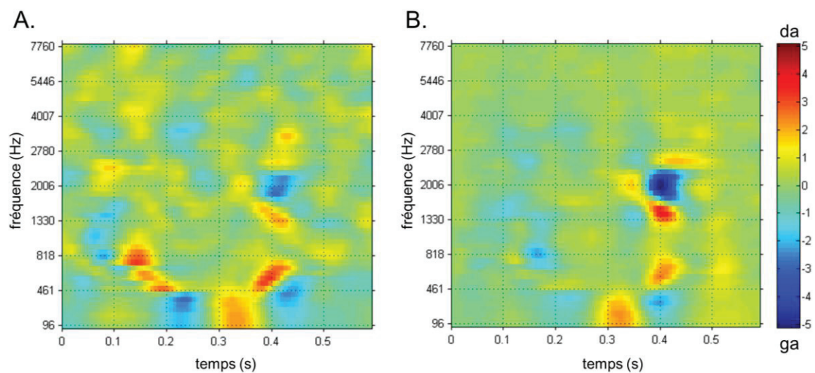
Figure 26 - ACIs moyennes pour la tâche de catégorisation /da/-/ga/. A. Expérience à 2 signaux (/alda/ et /alga/) (N=3 participants). B. Expérience à 4 signaux (/alda/, /alga/, /aɪda/ et /aɪga/) (N=19 participants).
