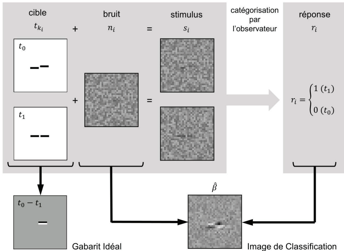
Figure 21 - Diagramme schématisé du paradigme expérimental employé pour le calcul des CIs. Les exemples de cibles, stimuli, gabarit idéal et la CI correspondante sont tirés de la tâche d'acuité de Vernier (Ahumada, 1996).
