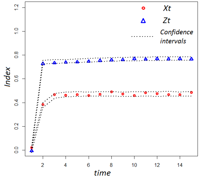
FIGURE II.2 – Modèle jouet II.17 : Indices estimés de Sobol en fonction du temps. Echantillon de taille : 10000. Intervalle de confiances à 95% en pointillé.
