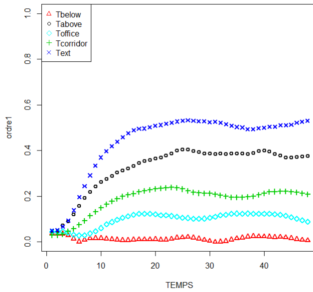
FIGURE III.1 – Indice de sensibilité en fonction du temps. Modèle E-A en entrée et entrée-sortie S1-A ( VARX )
