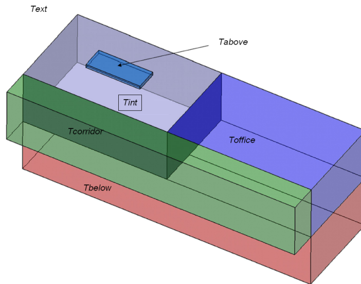
FIGURE III.1 – Agencement des différentes pièces
