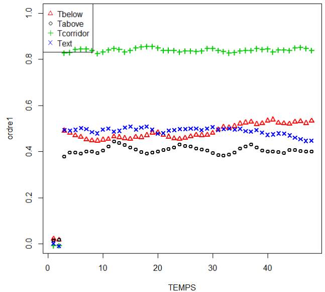
FIGURE III.3 – Indice de sensibilité en fonction du temps. Modèle E-B en entrée et modèle de sortie S2-B (regression)
