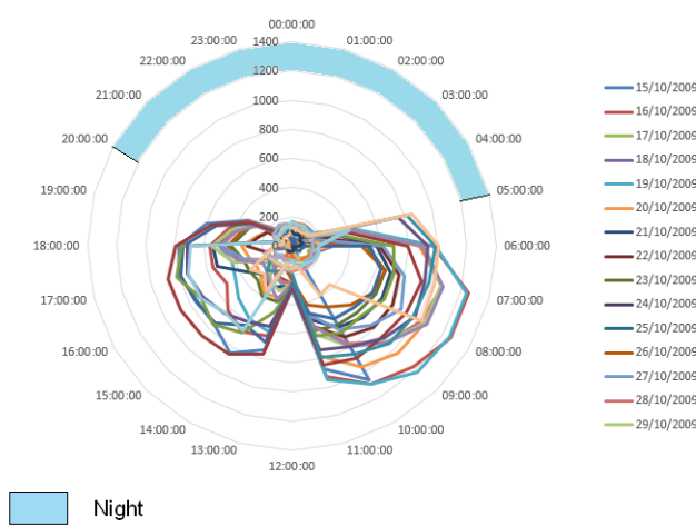
FIGURE III.7 – Représentation sur une journée du chauffage en Watt du 15/10/2009 au 15/11/2009
