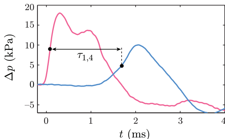
Figure 5.11 – Signaux de pression enregistrés aux capteurs 1 et 4 pour une fraction liquide de 8 % et une taille de bulles de 95 \mu\text{m} . Les deux cercles pleins indiquent la valeur à mi-hauteur de la pression sur chaque signal. Le délai entre ces deux points est alors \tau_{1,4} .
