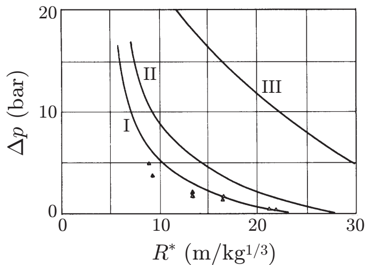
Figure 2.8 – Surpression en fonction de la distance réduite (distance réelle divisée par la masse de la charge à la puissance 1/3 ). I - Résultats obtenus dans une mousse dont la phase gazeuse est du dihydrogène. II - Résultats obtenus lorsque la phase gazeuse est du diazote. III - Courbe témoin représentant la décroissance de la surpression lors d'une explosion dans l'air. Figure extraite de [ Borisov et al. , 1978 ].
