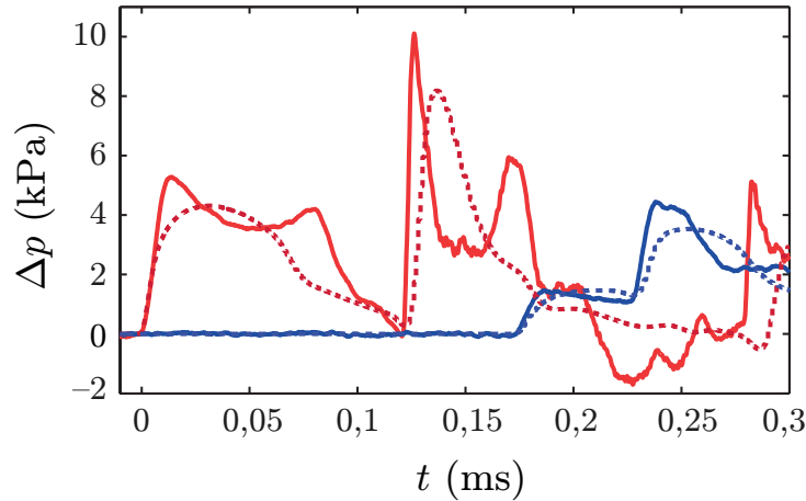
Figure 3.20 – Comparaison des signaux obtenus expérimentalement (trait plein) et par simulation numérique (trait pointillé) aux capteurs 1 et 4. L'entrefer est de 3 cm.
