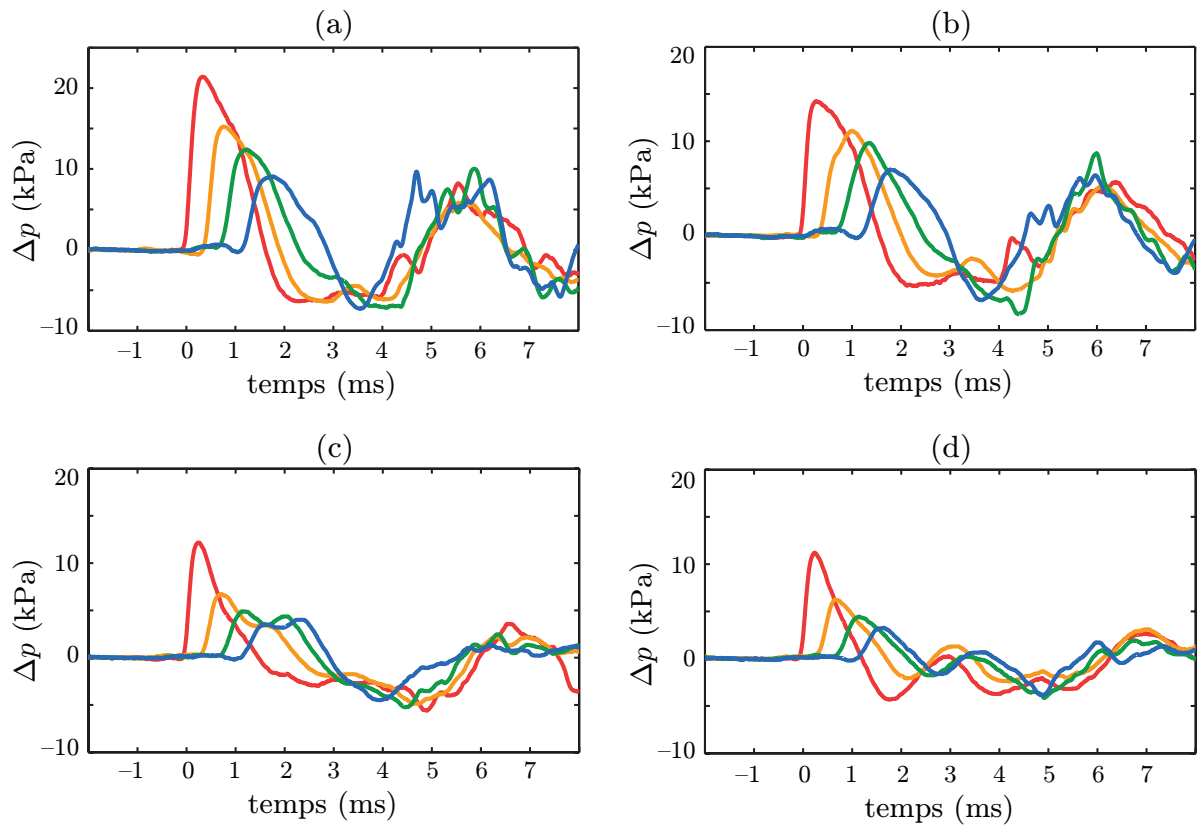
Figure 3.29 – Signaux de pression enregistrés dans la mousse après le passage de l’onde pour différentes valeurs de l’entrefer : H = 1,7 cm (a), H = 3 cm (b), H = 5 cm (c) et H = 8 cm (d). Les différentes couleurs correspondent aux différents capteurs.
