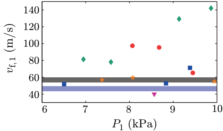
Figure 5.22 – Vitesse de l'onde v_{f,1} , mesurée au capteur 1, en fonction de l'amplitude du choc P_1 à ce même capteur, dans la limite des basses amplitudes ( P_1 \lesssim 10 kPa). Les rectangles bleu et noir indiquent respectivement les vitesses de Wood isotherme et adiabatique, avec leur incertitude liée à la fraction liquide. Les conventions adoptées pour les couleurs et les symboles sont identiques à celles définies sur la Figure 5.15.
