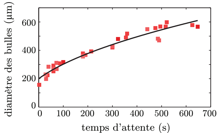
Figure 3.8 – Tailles de bulles en fonction du temps d’attente. Les carrés sont les points expérimentaux, obtenus avec le mélange turbulent, et la courbe noire est un ajustement de la forme d_0 \sqrt{1 + t/t_c} , avec d_0 et t_c laissés comme paramètres ajustables. Nous avons ici d_0 \approx 200 \mu\text{m} et t_c \approx 80 \text{ s} .
