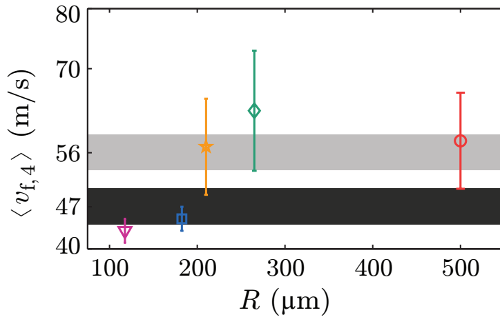
Figure 5.17 – Vitesse de front moyennée \langle v_{f,4} \rangle en fonction de la taille des bulles, pour des surpressions P_4 \lesssim 10 kPa. Les rectangles noirs et gris représentent respectivement les vitesses de Wood isotherme et adiabatique avec une barre d’erreur provenant de celle sur la fraction liquide.
