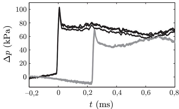
Figure 3.17 – Superposition de 3 signaux de chocs, chacun obtenu avec 3 feuilles d'aluminium en guise de diaphragme, illustrant la bonne reproductibilité de notre montage expérimental.
