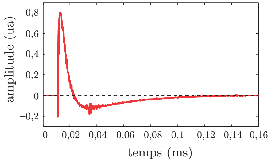
Figure 3.10 – Profil de surpression généré dans l'air par l'explosion d'un pétard à mèche. La dépression à t = 0 est un artefact très probablement lié au temps de réponse du micro.
