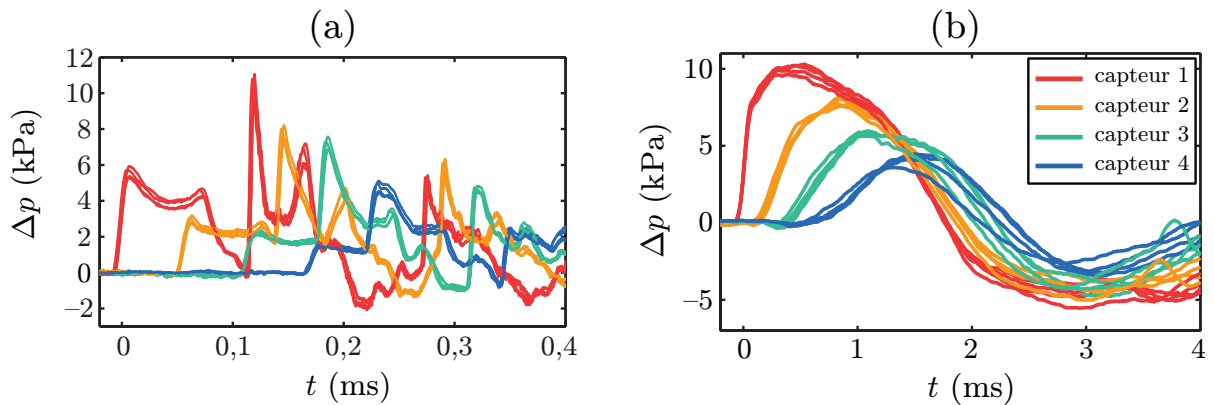
Figure 3.21 – Superposition de 4 séries de signaux de pression mesurés dans l'air (a) et dans la mousse (b) lors du passage du soufflé entre les plaques illustrant la bonne reproductibilité des tirs avec le tube à choc. L'entrefer est de 3 cm et une feuille d'aluminium a été utilisée en guise de diaphragme dans le tube à choc.
