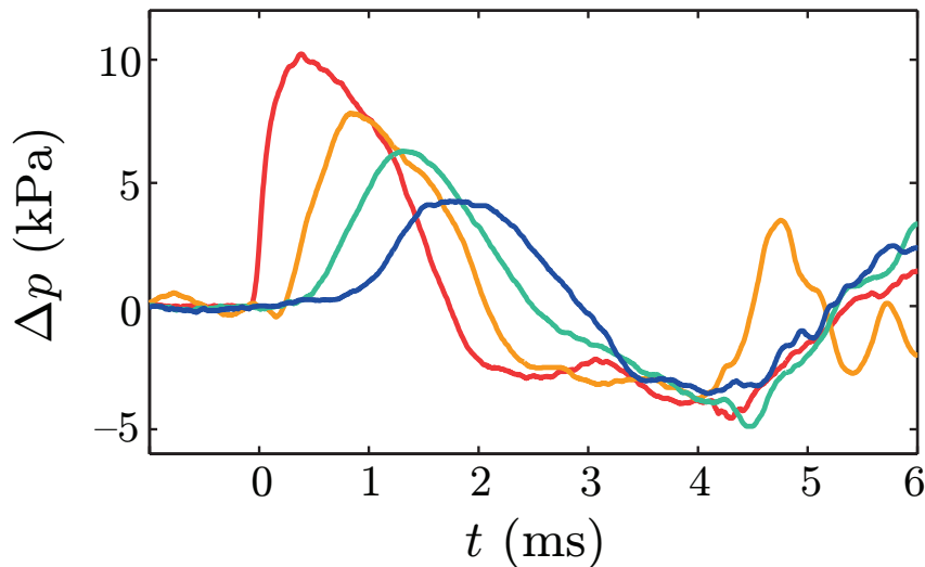
Figure 6.5 – Exemple de signaux de pression bruts enregistrés (ici pour une taille de bulles de 210 \mu\text{m} ). Les pics secondaires arrivant à 4 ms correspondent au retour de l'onde réfléchi sur le bord extérieur de la mousse.
