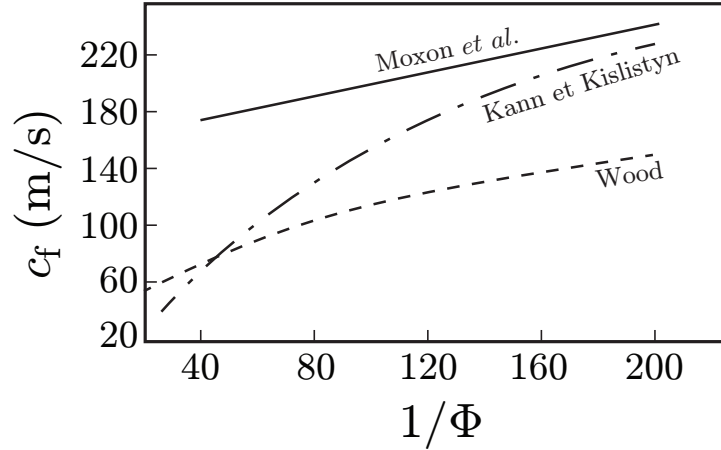
Figure 1.11 – Vitesse du son dans une mousse en fonction de l’inverse de la fraction liquide. En trait plein, les données expérimentales de Moxon et al. , la courbe en pointillés alternés représente le modèle de Kann et Kislitsyn et la courbe en pointillé régulier correspond au modèle de Wood. Figure extraite de [Kann et Kislitsyn, 2003].
