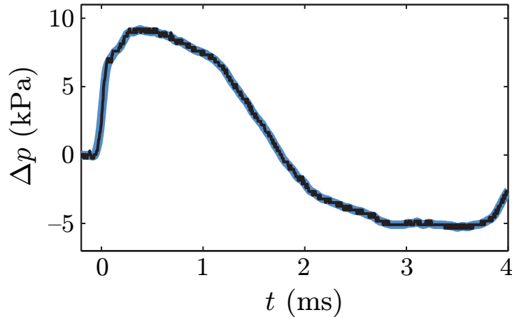
Figure 3.22 – Signal de pression mesuré dans une mousse. En noir : signaux bruts. En bleu : signaux lissés sur 15 points, soit sur 0,06 ms environ.
