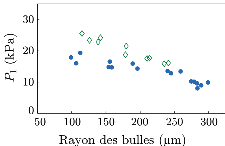
Figure 3.23 – Amplitude du premier pic de pression dans la mousse en fonction de la taille des bulles lorsque l’on utilise une feuille d’aluminium (●) ou deux (◇). Les points expérimentaux ont été obtenus avec le mélange turbulent.
