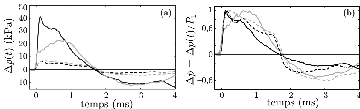
Figure 3.24 – (a) Signaux de pression bruts au capteur 1 pour des bulles de 120\ \mu\text{m} (en noir) et de 265\ \mu\text{m} (en gris). Les courbes en trait plein sont obtenues avec un diaphragme de 4 feuilles d’aluminium, celles en trait pointillé avec une feuille de parafilm. (b) Signaux renormalisés par l’amplitude du pic.
