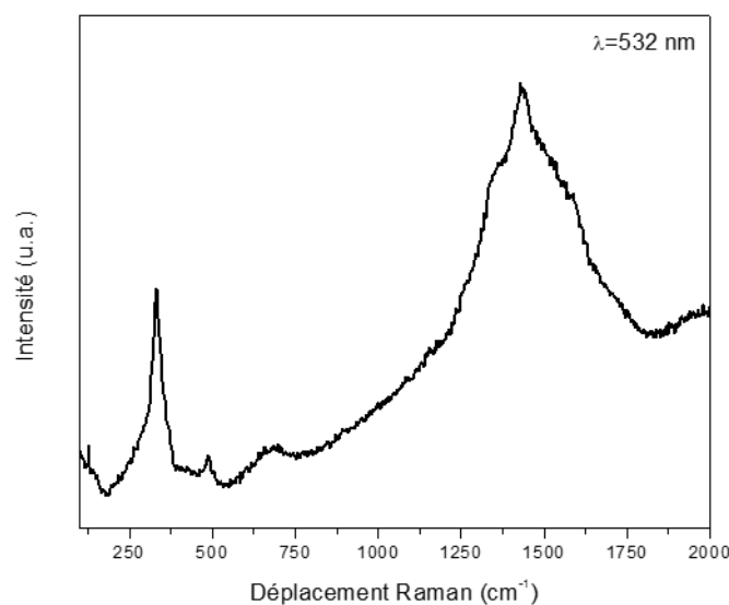
FIGURE 6.18: Spectre Raman d'une couche mince séchée à 400\text{ °C}
