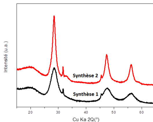
FIGURE 4.20: Diffractogrammes de poudres obtenues par synthèse en réacteur continu séchées à 300 °C pour deux compositions différentes
