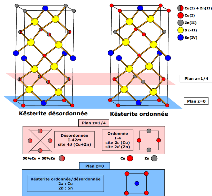
FIGURE 1.8: Mailles cristallines des phases kèsterite et kèsterite désordonnée [25]
