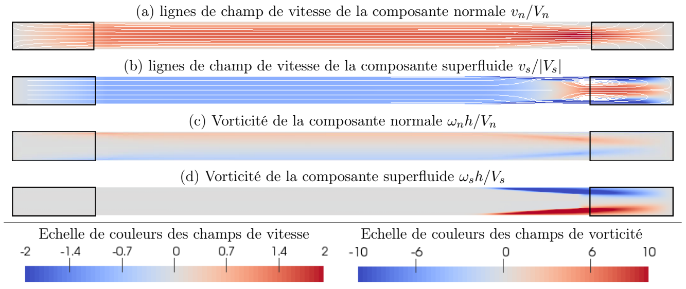
FIGURE 3.3: Lignes de champ de vitesse et champs de vorticité pour une simulation de contre-courant à 1,5 K avec couplage HVBK. Les paramètres de la simulation sont regroupés dans les tableaux 3.2, 3.3 et 6.2 (en annexe). Les contours noirs symbolisent les limites du thermostat chaud et du thermostat froid.
