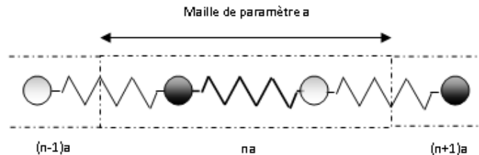
Figure 2-1 : Représentation de la chaîne linéaire à deux atomes par maille.
