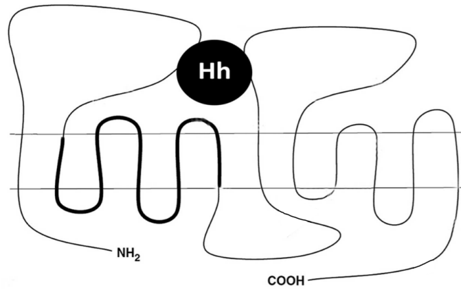
Figure 13 : Structure de la protéine PTCH1 . On retrouve les 12 domaines transmembranaires et les deux grosses boucles extracellulaires nécessaires à l'interaction avec le ligand hedgehog. Le trait gras correspond au domaine sensible aux stérols (SSD). D'après Yu et al. (90).
