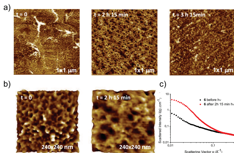
Figure A5 | Caractérisations micro- et nanoscopiques du gel 6 (PEG 5000). a) Images AFM du gel 6 soumis à différents temps d'irradiation UV: avant contraction ( t = 0 ), après contraction ( t = 2 \text{ h } 15 \text{ min} ), et après éclatement du gel ( t = 3 \text{ h } 15 \text{ min} ). b) Images AFM détaillées avant et après contraction du gel 6 mettant en évidence l'augmentation de la taille moyenne des pores du gel de 8 nm à 20 nm. c) Données obtenues par diffusion des rayons X aux petits angles avant et après irradiation du gel 6 .
