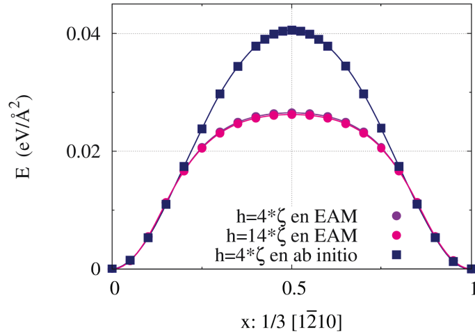
FIGURE 3.2 – Influence de la hauteur h de boîte de simulation sur l'énergie de faute d'empilement dans le plan pyramidal \pi_{1L} pour un vecteur faute colinéaire au vecteur 1/3[\bar{1}210] . Les points correspondent aux résultats des simulations atomiques et les lignes à leur interpolation en série de Fourier.
