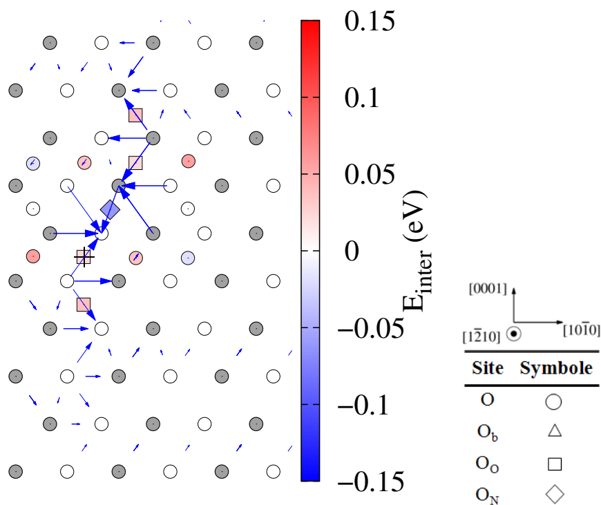
FIGURE 5.12 – Énergie d'interaction entre l'oxygène et la dislocation vis pyramidale métastable calculée pour différentes positions de l'atome d'oxygène. L'énergie illustrée par un dégradé de couleur rouge et bleu est superposée à la carte de Vitek de la dislocation dans sa configuration métastable pyramidale. Les énergies d'interaction sont calculées par rapport à la configuration métastable.
