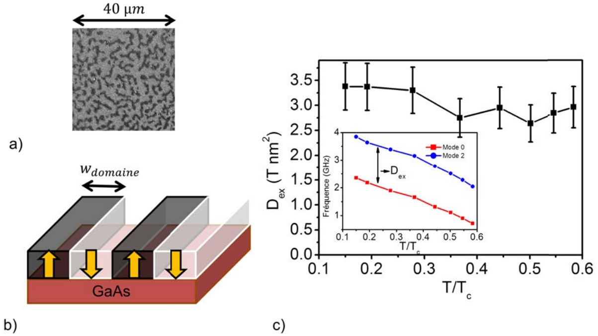
Figure 9.8: a : Image obtenue en microscopie Kerr sur l'échantillon de l'équipe de Nemec et al. ( \text{Mn}_6\text{P}_{10} ) ayant servi dans [183] à T=95 K ( T/T_c = 0.86 ). b : Schéma représentant l'organisation à T=95 K. c : D_{ex} en fonction de la température normalisée par la T_c (=85 K) mesuré en TRMOKE sur \text{Mn}_7\text{P}_{4.3} . En encart est représentée l'évolution des fréquences de précession en fonction de la température normalisée par T_c .
