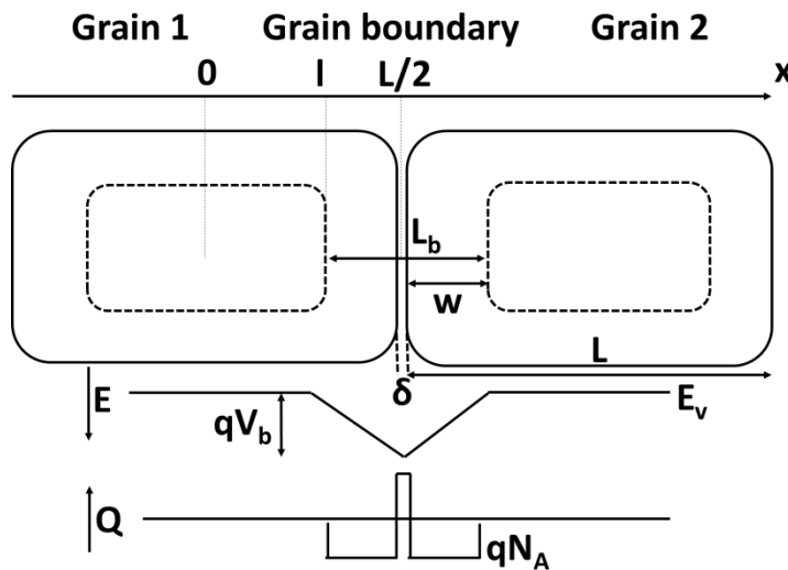
Figure II.5. Représentation schématique du transport dans le poly-Si. Les rectangles représentent les grains, en pointillés les zones de déplétion de largeur w . En dessous sont représentées la variation d'énergie de la BV et la distribution de la charge dans les grains et GBs. L'origine de l'axe x se trouve au centre d'un GB et l représente la distance entre le centre d'un grain et le bord de la zone de déplétion.
