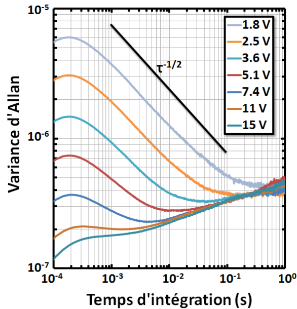
Figure V.28. Variance d'Allan en fonction du temps d'intégration pour différentes tensions (AC) d'alimentation. On peut constater la diminution du bruit blanc en fonction de l'alimentation.
