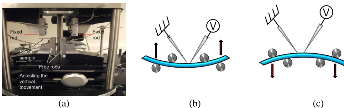
Figure III.1. (a) Photo du banc de mesure quatre points sous contrainte mécanique « four-points-bending test » du CEA-LETI. (b) et (c) sont des représentations schématiques d'une mesure avec une contrainte en compression (b) et en tension (c). Cette contrainte est maintenue grâce à quatre supports, deux fixes et deux amovibles. Une relation liant le déplacement des supports et leur position horizontale permet de connaître la contrainte appliquée.
