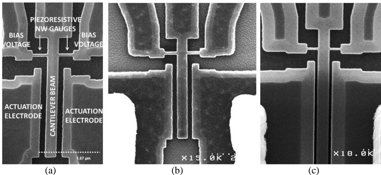
Figure 2. Photos SEM du NEMS cross-beam avec une couche active de : poly-Si « chaud » (a), « froid » (b) et c-Si (c).
