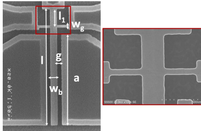
Figure V.1. (a) Photo SEM du NEMS cross-beam. L'encadré rouge (b) permet d'observer les jauges nanofils de contrainte de 80 nm de largeur.
