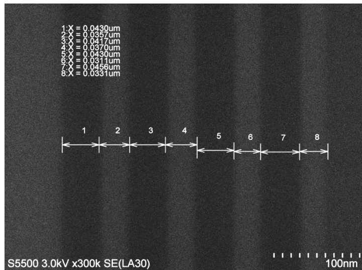
Figure IV.42. Photo SEM en coupe de l'empilement 4×SiO 2 (zones sombres)/ SiN (zones claires). Les épaisseurs de chaque couche ont été extraites.
