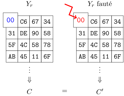
FIGURE 4.6 – Exemple de faute sans effet
