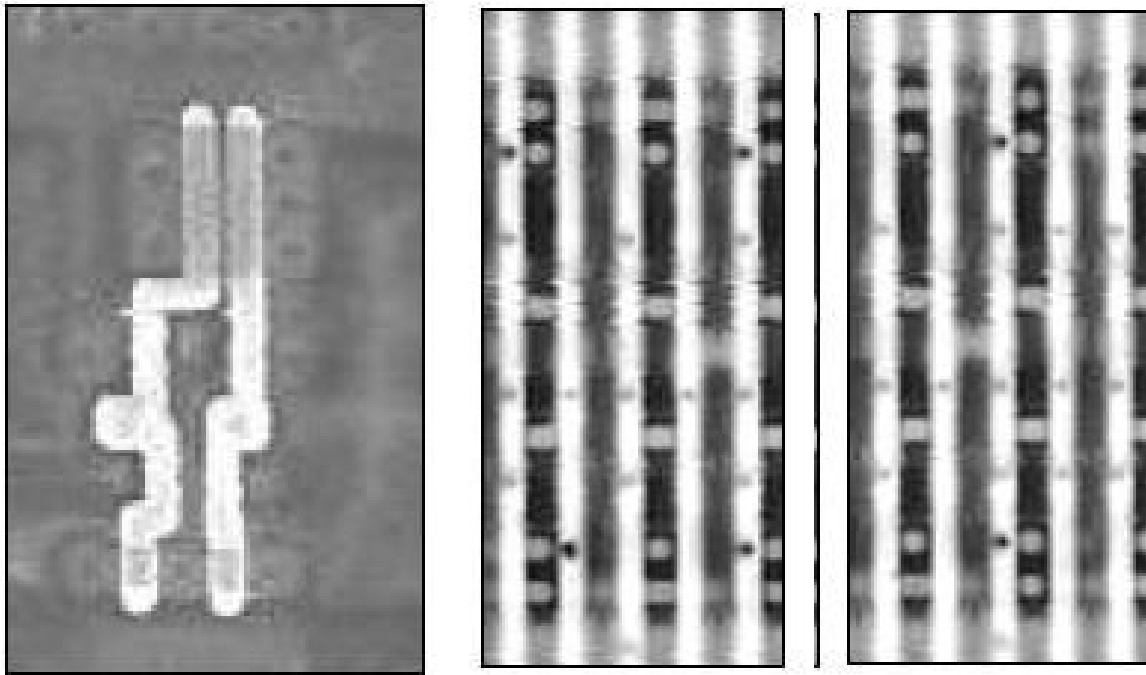
FIGURE 5.1 – Camouflage bas niveau de portes logiques. Gauche : porte logique non protégée dont la fonction peut être identifiée visuellement. Milieu, droite : Portes logiques ET et OU pratiquement indistinguables visuellement. [avec l'aimable autorisation de SMI / SypherMedia Library]
