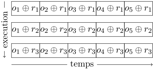
FIGURE 1.13 – Illustration de la contre-mesure utilisant des masques
