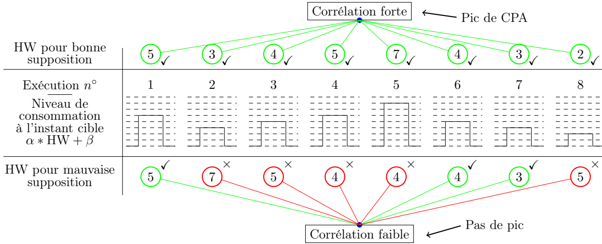
FIGURE 1.9 – Shématisation de la méthode CPA : Obtention d'un pic de CPA pour la bonne supposition de valeur de clé (en haut) et non-obtention d'un pic lors des mauvaises suppositions (en bas)
