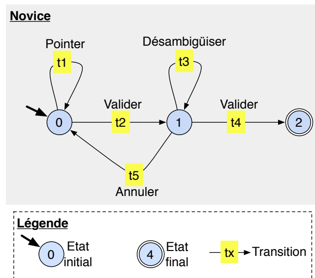
FIGURE 5.2 – Automates de nos techniques illustrant le comportement attendu d'utilisateurs novices.
