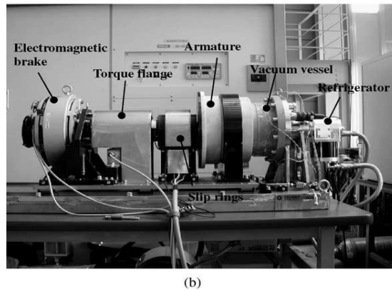
Figure 20 : a) la structure du moteur et b) une photographie de l'expérience de M. Hirakawa et al.
