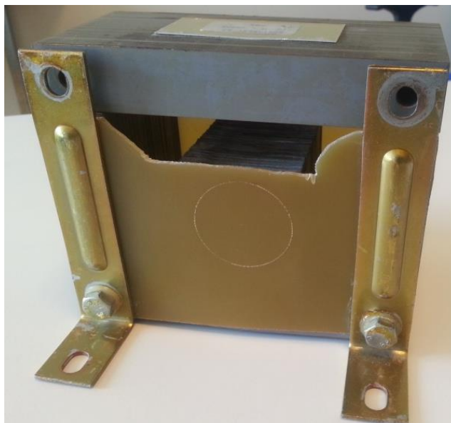
Figure 78 : Circuit magnétique réalisé.
