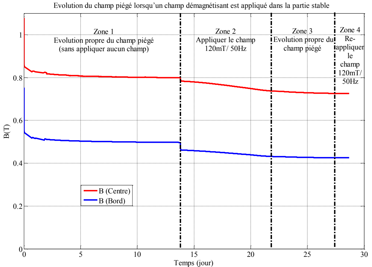
Figure 103 : Évolution du champ piégé lorsqu'un champ démagnétisant AC 120 mT /50 Hz est appliqué dans la partie stable (après 5 jours).
