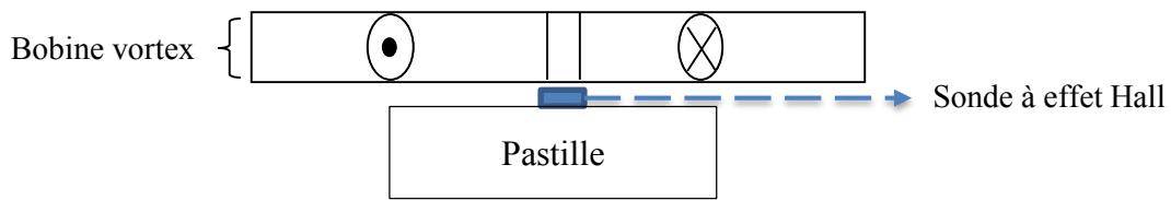
Figure 44 : Représentation du système d'aimantation par la bobine vortex.
