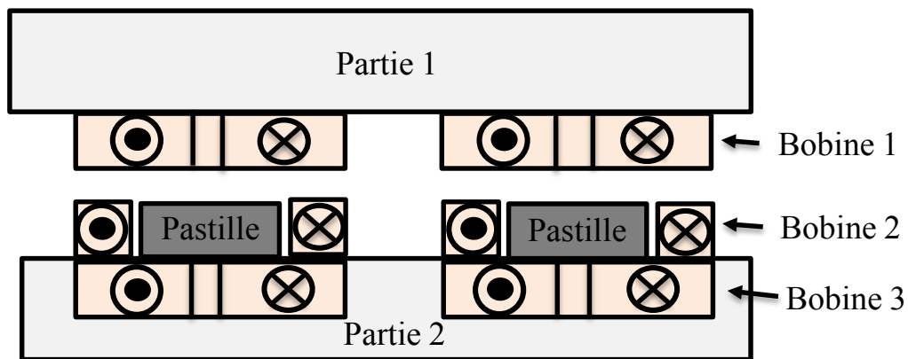
Figure 118 : Accouplement magnétique en utilisant des pastilles supraconductrices aimantées.
