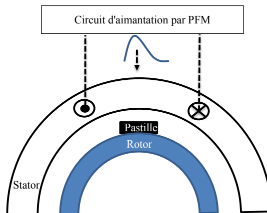
Figure 32 : Aimantation par le stator d'une pastille placée sur le rotor d'un moteur électrique.
