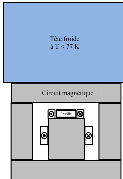
Figure 116 : Étude à basse température dans un circuit magnétique.
