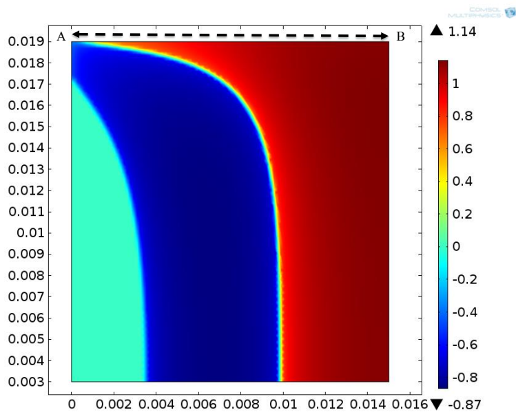
Figure 94 : Distribution de J/J_c dans une pastille aimantée par une petite impulsion en pénétration incomplète.
