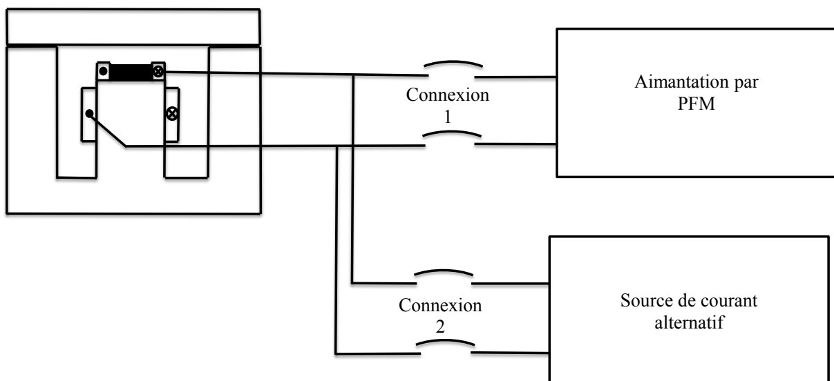
Figure 99 : Schéma des connexions électriques de l'expérience concernant l'effet d'un champ démagnétisant alternatif.
