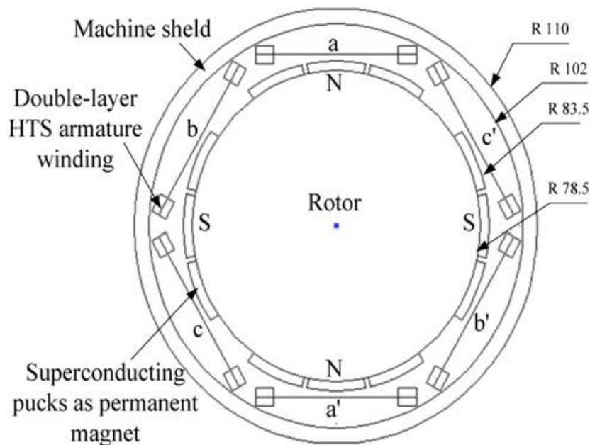
Figure 21 : Structure générale du moteur proposé par Y Jiang et al.
