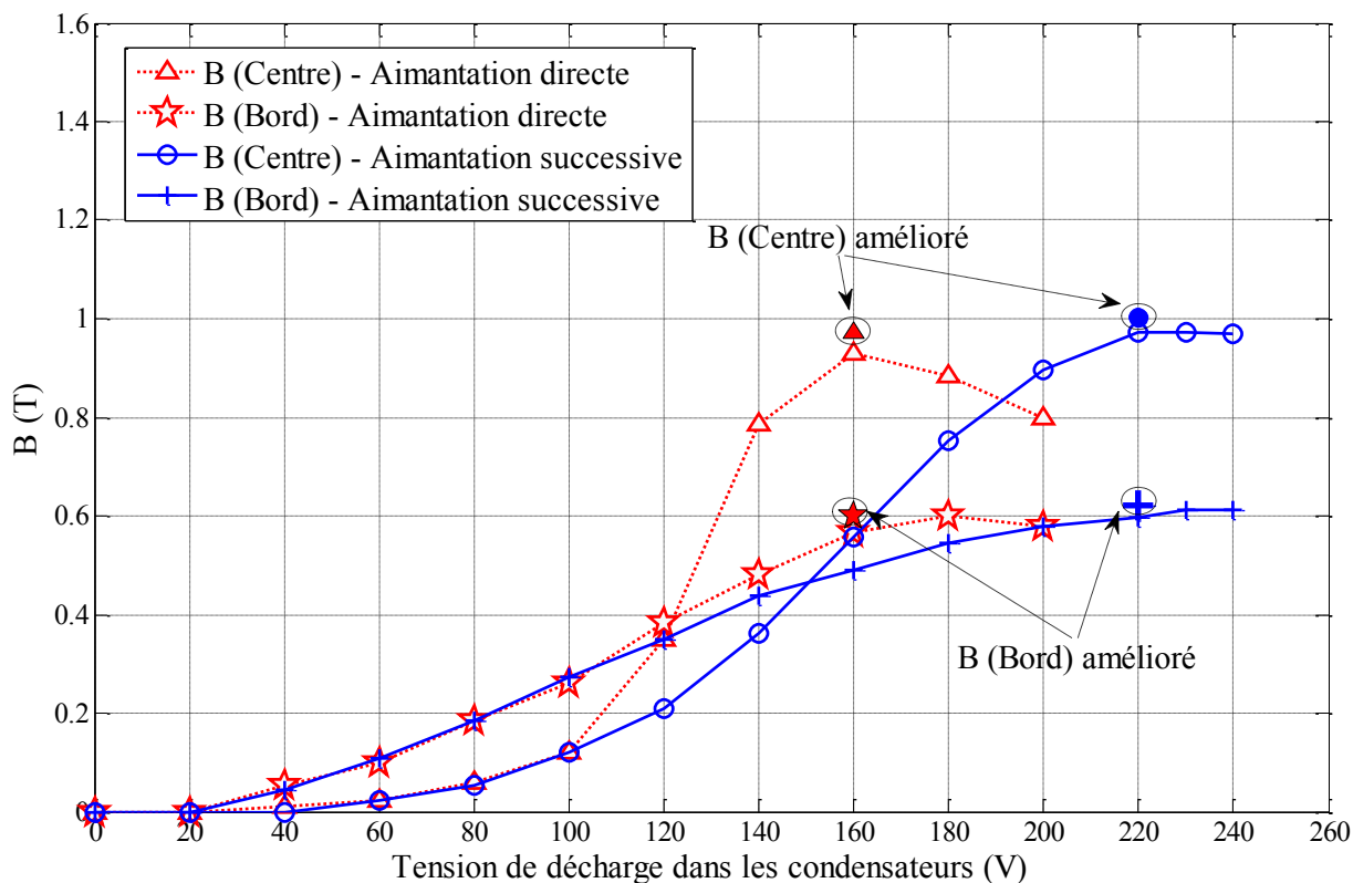
Figure 92 : Comparaison des champs piégés en fonction de la tension de décharge des condensateurs pour les procédés d'aimantation direct et successif et leur version améliorée.
