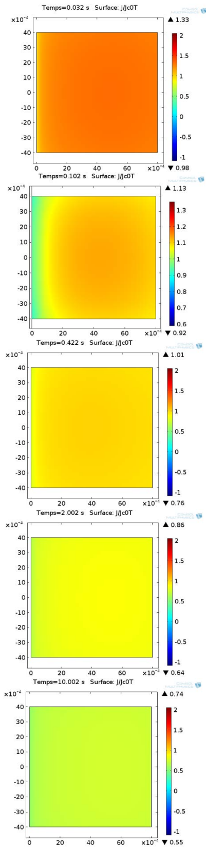
Figure 62 : Evolution de la température après la fin de l'impulsion et son effet sur la densité de courant.
