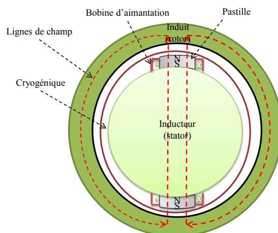
Figure 64 : Schéma d'une machine synchrone avec des pastilles supraconductrices.
