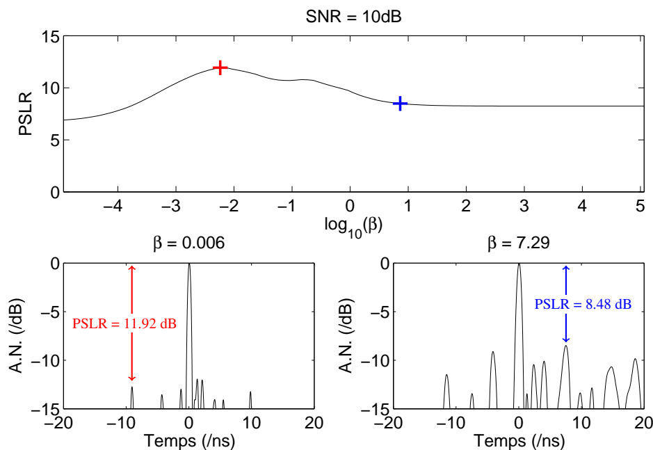
FIGURE 2.29 – Détermination du PSLR pour un SNR = 10 dB et un pointage dans la direction \theta = -20^\circ . Le calcul est effectué pour un ensemble de valeurs de \beta régulièrement espacées dans la plage de variation [10^{-5}, 10^5] . La figure supérieure présente la variation du PSLR en fonction de \beta . Deux exemples de mesures sont extraits pour des valeurs différentes de paramètre de régularisation.
