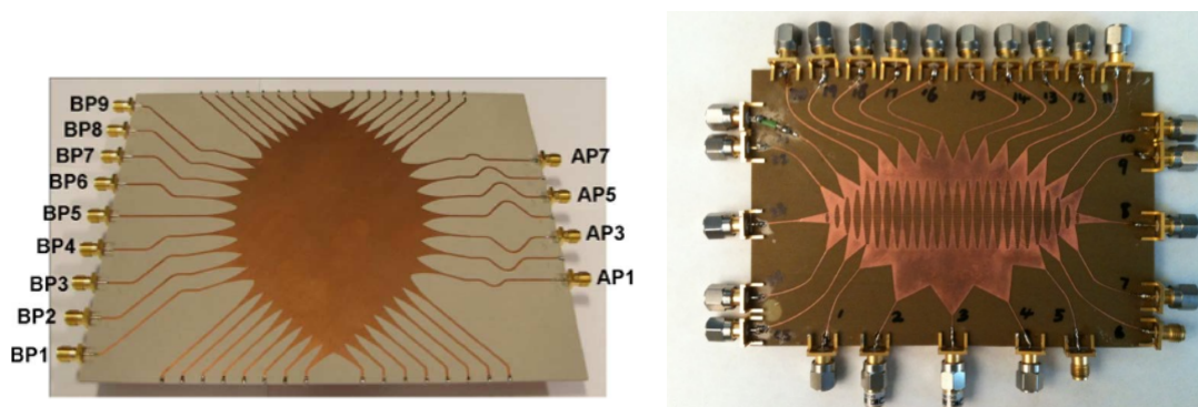
(a) Lentille de Rotman conventionnelle [17]. (b) Lentille compressée par l'utilisation de métamatériaux [18].
