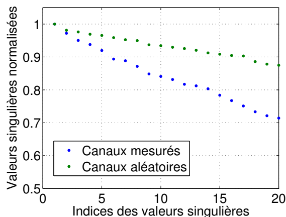
FIGURE 4.10 – Spectre de valeurs singulières de la matrice de fonctions de transfert mesurée, comparée à une matrice aléatoire de dimensions identiques.
