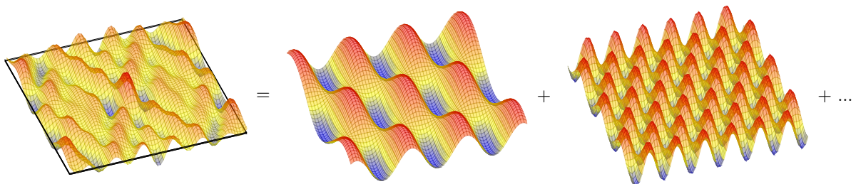
FIGURE 2.4 – Décomposition modale du champ établi dans la cavité à une fréquence
