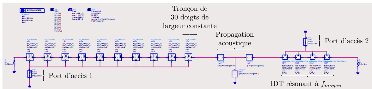
FIGURE 3.12 – Modèle circuit d'un filtre SAW OFC simulé avec ADS .
