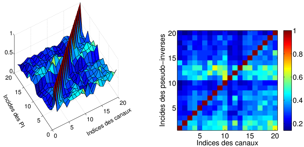
FIGURE B.4 – Niveaux de corrélations calculés entre les fonctions de transfert mesurées et les pseudo-inverses correspondants obtenus par régularisation de Tikhonov.
