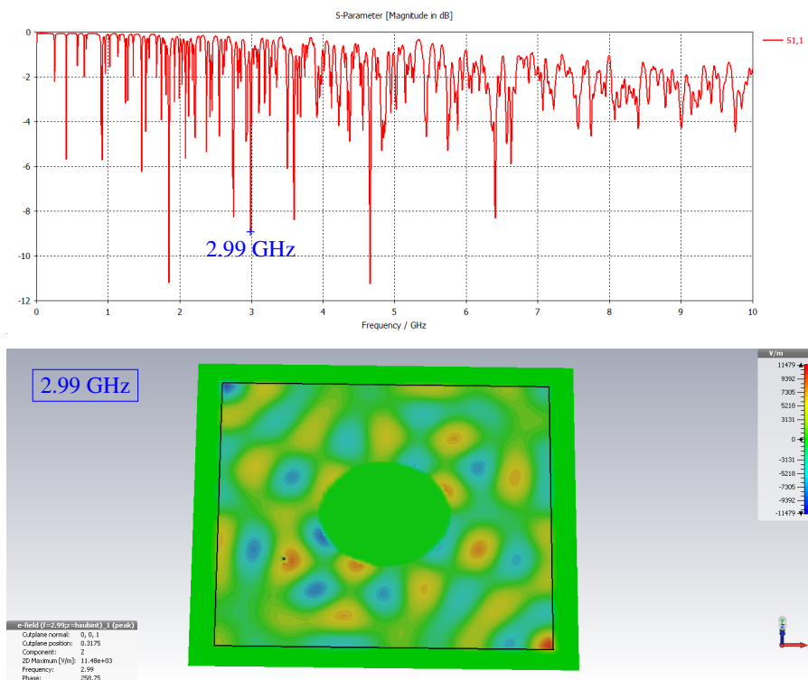
FIGURE 2.56 – Coefficient de réflexion de la cavité chaotique 2D simulée sous CST et représentation des modes établis à une fréquence.
