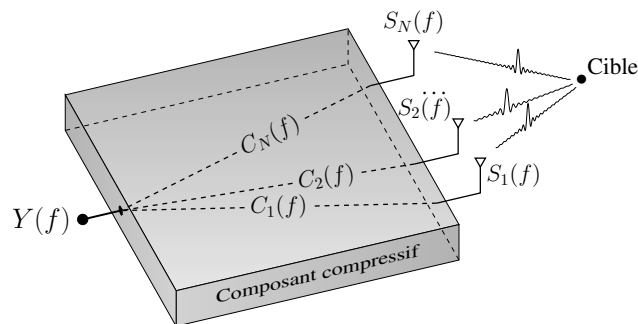
FIGURE 1.25 – Représentation de la compression des ondes reçues par un réseau d'antennes en un signal unique. Ce composant réalise ainsi un multiplexage des signaux reçus par l'utilisation de canaux orthogonaux.
