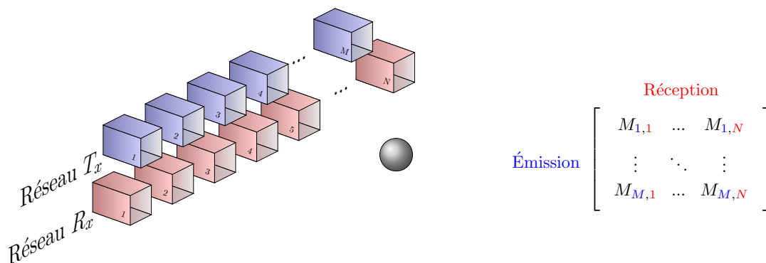
FIGURE 4.1 – Système bistatique linéaire et matrice d'interaction équivalente
