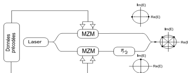
Figure I. 21. Structure d'un Emetteur DQPSK.
