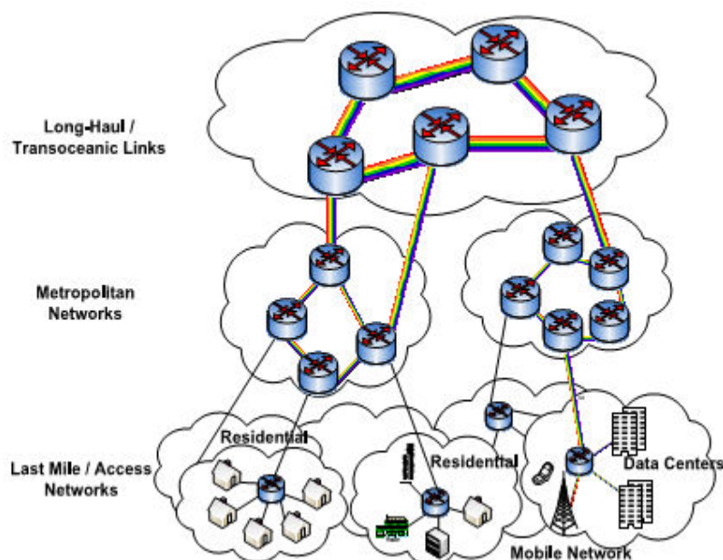
Figure I. 1 –Schématisation d’architecture d’un réseau optique.
