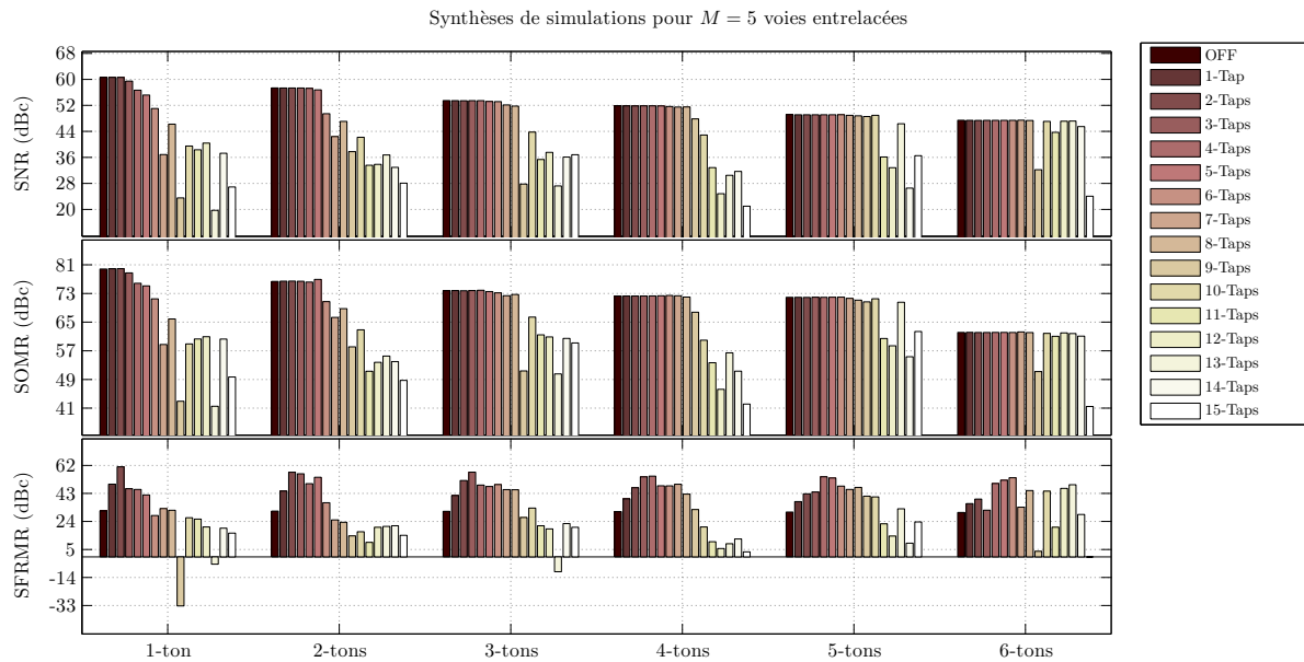
FIGURE G.4 – Synthèse de simulation de l'architecture de compensation adaptative pour M = 5 voies entrelacées et des disparités de gains, de décalages temporels et de bandes passantes.
