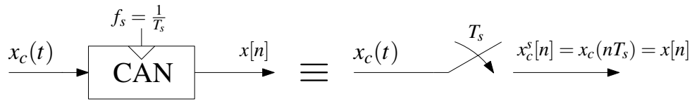
FIGURE 2.1 – Modèle simplifié de la conversion par un CAN du signal analogique x_c(t) à la fréquence d'échantillonnage f_s donnant le signal numérique x[n] .
