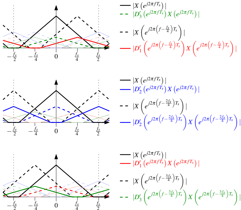
FIGURE 3.2 – Représentation pour M = 4 des modules en fréquence du signal avec les disparités de réponses fréquentielles, présenté dans la Figure 2.14, puis de ses 3 translatés en fréquence de \eta \frac{f_s}{4} avec \eta \in \{1, 2, 3\} et enfin les 3 corrélations entre le signal avec les disparités et chacune de ses translatés en fréquence.
