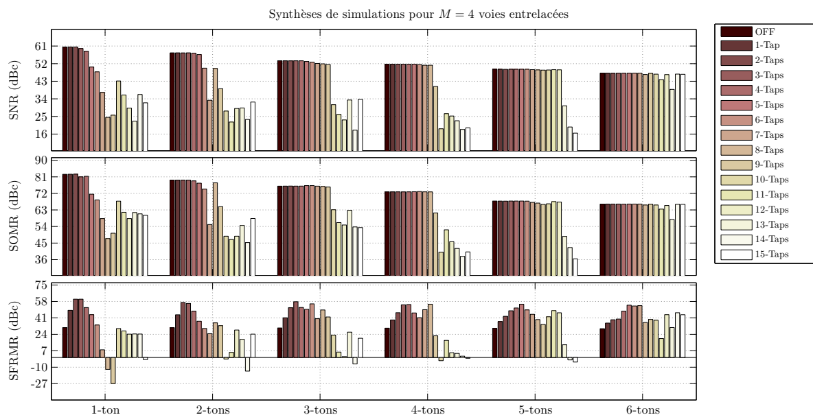
FIGURE 4.20 – Synthèse de simulation de l’architecture de compensation adaptative pour M = 4 voies entrelacées et des disparités de gains, de décalages temporels et de bandes passantes.
