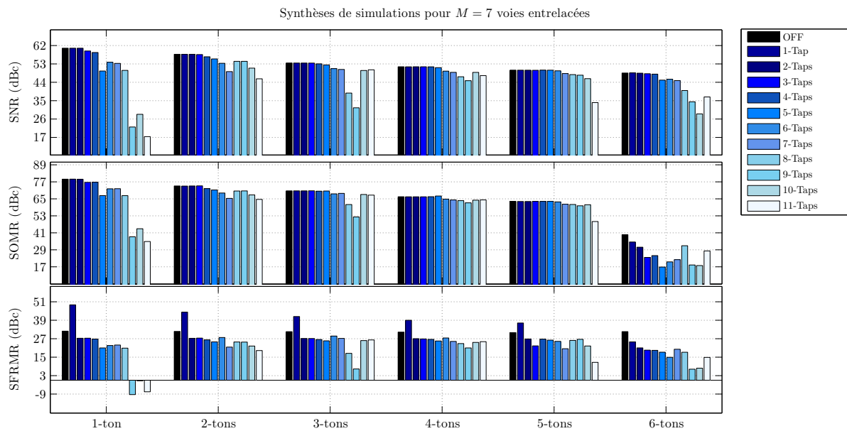
FIGURE G.3 – Synthèse de simulation de l'architecture de compensation direct pour M = 7 voies entrelacées et des disparités de gains, de décalages temporels et de bandes passantes.
