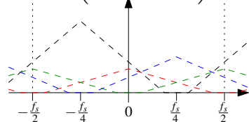
FIGURE 3.2 – Représentation pour M = 4 des modules en fréquence du signal avec les disparités de réponses fréquentielles, présenté dans la Figure 2.14, puis de ses 3 translatés en fréquence de \eta \frac{f_s}{4} avec \eta \in \{1, 2, 3\} et enfin les 3 corrélations entre le signal avec les disparités et chacune de ses translatés en fréquence.
