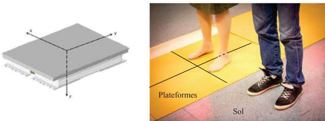
Figure 16 : Chaque plateforme (schéma à gauche) enregistre les actions mécaniques entre le sol et le système qui vient en appui dessus. Dans le cadre de l'expérimentation (à droite), les quatre plateformes (séparée par les lignes noires pour l'illustration) étaient intégrées au sol.
