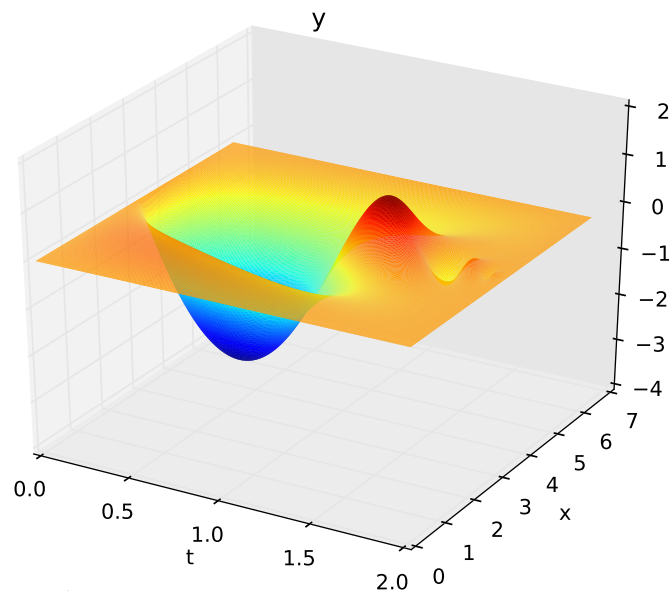
FIGURE V.2: Évolution de la composante y du système (3.1) dans le cas (a).
