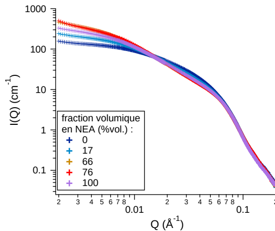
Fig. II.24 : Diffractogrammes obtenus par SAXS pour des échantillons de nanoparticules S recouvertes de PAA 2k pour différentes compositions de solvant NEA : eau. Les échantillons ont été obtenus par mélange d'une dispersion aqueuse à pH = 7,5 et d'une dispersion dans le NEA à pH = 8,2, toutes deux de fraction volumique égale à 0,1 %vol. en nanoparticules. Les courbes obtenues pour 66 et 76 %vol. apparaissent superposées.
