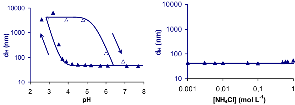
Fig. I.11 : Diamètre hydrodynamique obtenu par DLS pour une dispersion ( \phi = 0,05 à 0,10 %vol.) de nanoparticules C2 recouvertes de PAA 2k à gauche : à différents pH (sans sel ajouté), à droite : à différentes forces ioniques (à pH compris entre 6,4 et 6,8). La ligne continue est un guide pour l'œil.
