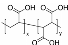
Fig. I.12 : Poly(acide acrylique-co-acide maléique)
