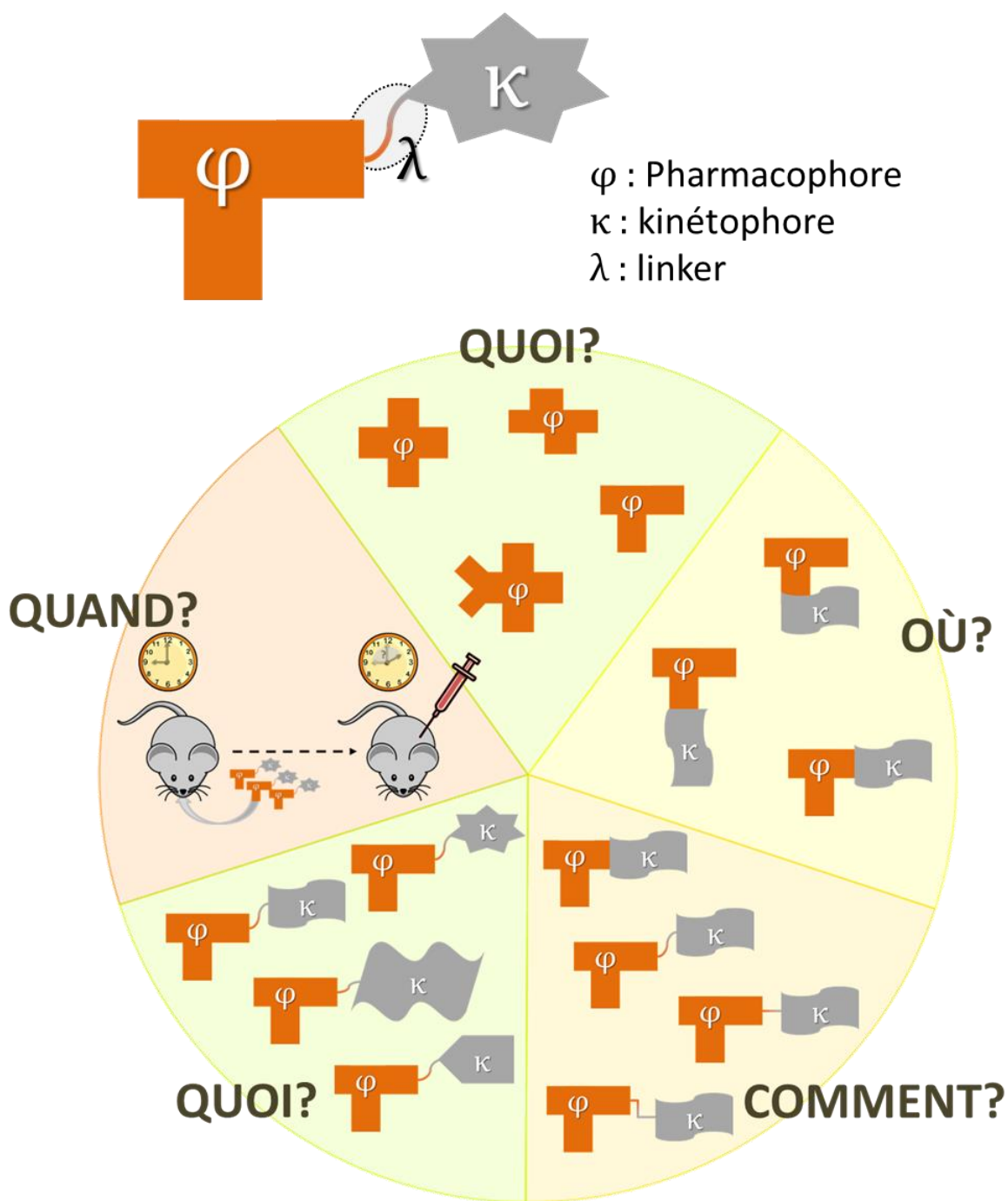
Figure 28 : Structure schématique d'un agoniste de TGR5 à visée topique intestinale et stratégie de développement.
