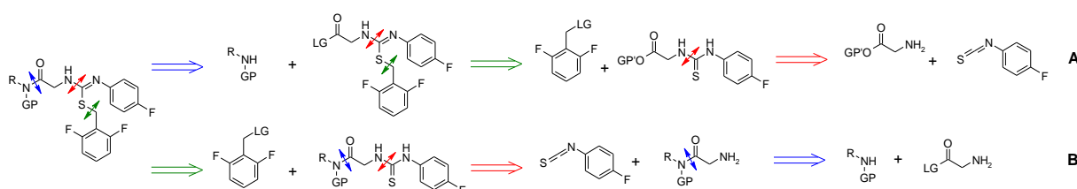
Schéma 21 : Modification de l'analyse rétrosynthétique de l'acétamidoisothiourée. La séquence du haut (analyse n°1bis, A) correspond à la nouvelle analyse envisagée. La séquence du bas ( B ) correspond à l'analyse ayant conduit à la voie de synthèse n°1.
