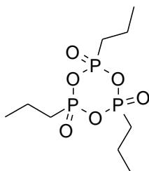
Figure 37 : Structure du T3P®.
