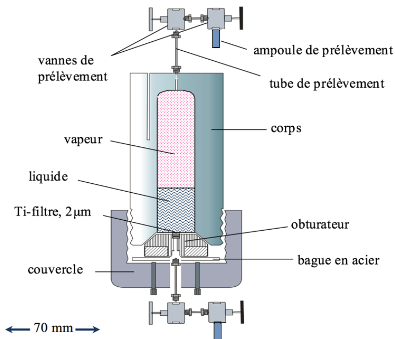
Fig. 2.2. Schéma du réacteur à séparation de phase ( T_{\max} = 360^{\circ}\text{C} , P_{\max} = 400 bar).
