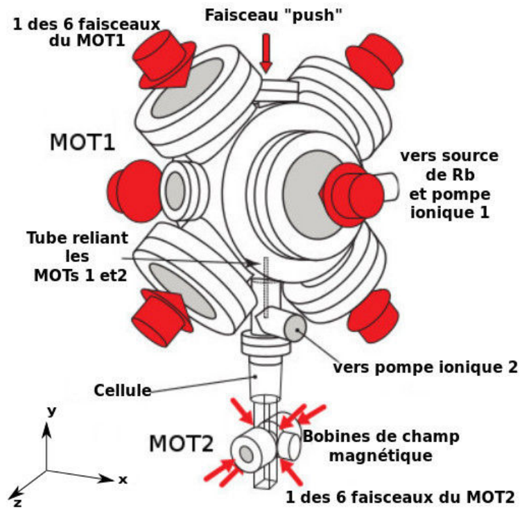
FIGURE 1.1 – Dispositif de l'expérience de BEC de ^{87}\text{Rb} à l'INLN. Source [5].
