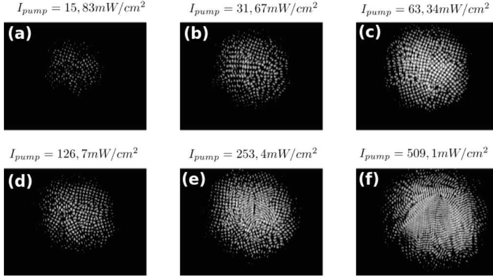
FIGURE 2.30 – Evolution des instabilités (dans le canal \perp ) en fonction de l'intensité de la pompe. Le désaccord du faisceau est \delta = -7,76 \Gamma et t_{pump} = 200 \mu\text{s} .
