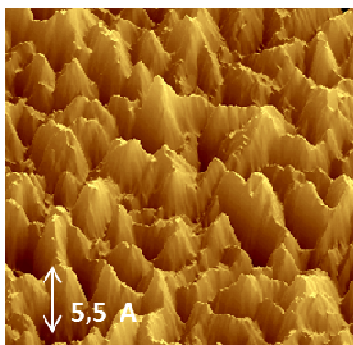
Figure III-16 : Topologie de surface du titane
