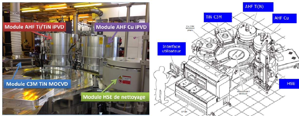
Figure III-2: Présentation des modules du réacteur Sigma 300 FxP®
