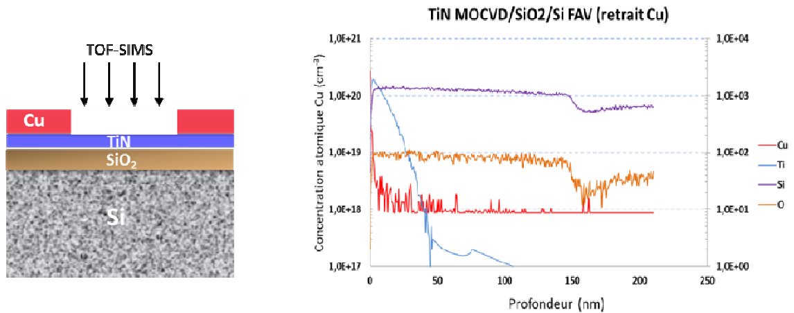
Figure IV-17: Mesure des propriétés barrière par TOF -SIMS avec retrait Cu
