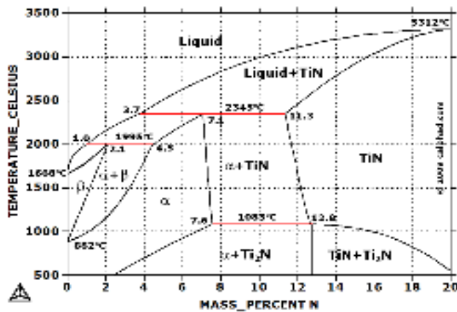
Figure III-30 : Représentation du diagramme de phase du nitrure de titane
