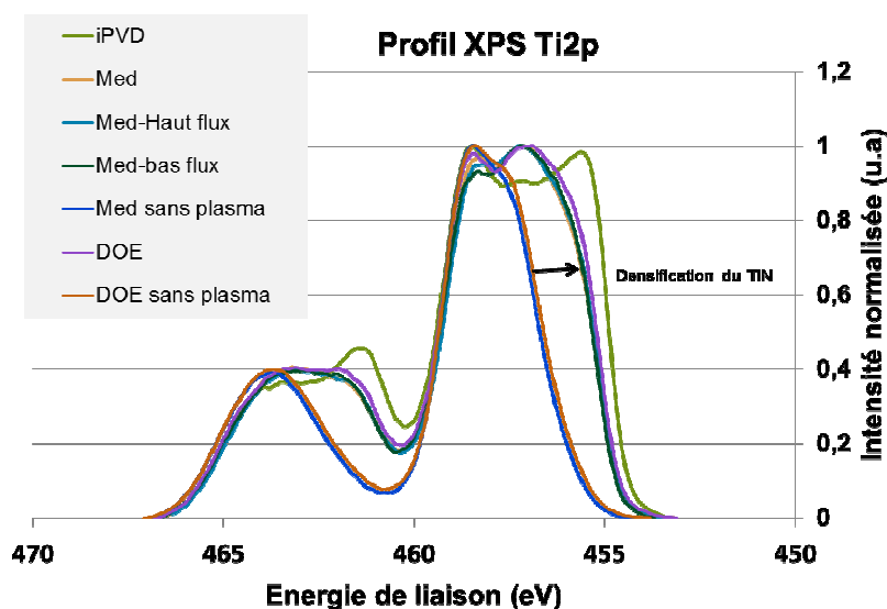
Figure III-43: Variation du spectre XPS de l'orbitale Ti2p
