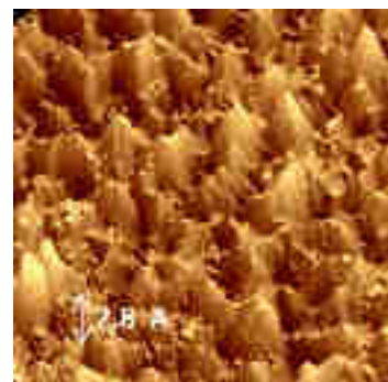
Figure III-21 : Topologie de surface du TiN à 160 sccm
