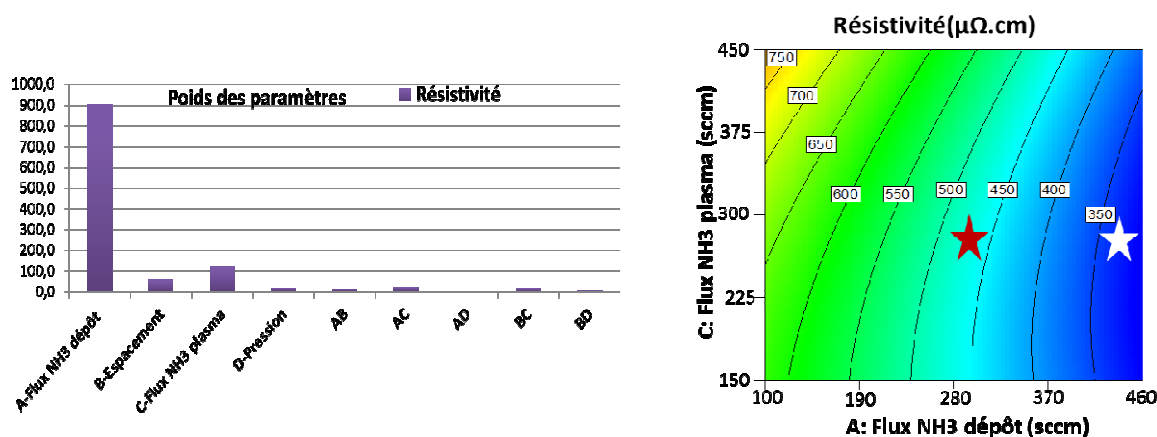
Figure III-41: Influence des paramètres sur la résistivité
