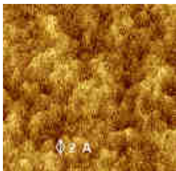
Figure III-19 : Topologie de surface du TiN à 120 sccm
