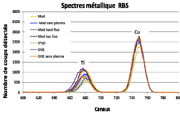
Figure III-48: Représentation du profil RBS des films
