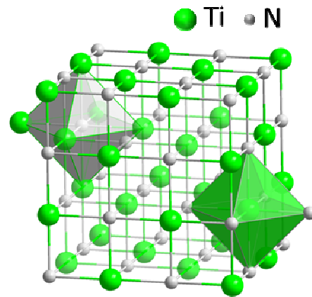
Figure III-31: Représentation de la structure CFC du nitrure de titane
