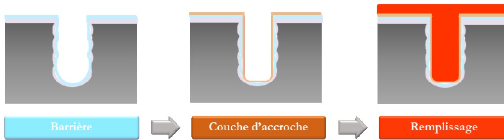
Figure I-28: Les étapes de la métallisation des vias
