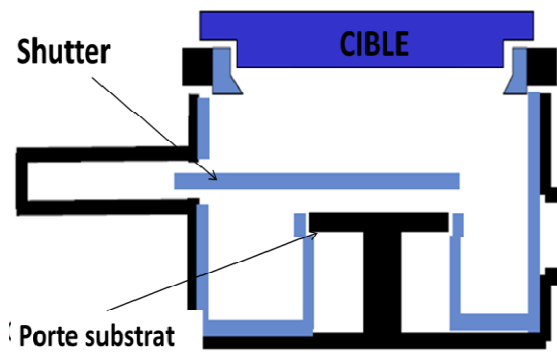
Figure III-4: Représentation du bâti de pulvérisation
