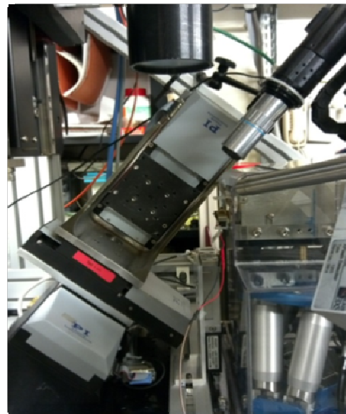
Figure IV-51 : Ligne BM32 de l'ESRF
