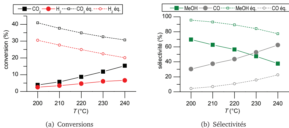
Figure 5.21 Effet de la température pour CuZZ à p_{\text{H}_2} = 34,9 bar, p_{\text{CO}_2} = 8,9 bar, p = 50 bar, \text{GHSV} = 7800 \text{ h}^{-1}
