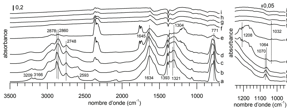
Figure 6.25 TPD d'acide formique du support ZC sous flux d'He suivie par DRIFTS (a) 100 °C, (b) 150 °C, (c) 200 °C, (d) 225 °C, (e) 250 °C, (f) 275 °C, (g) 300 °C, (h) 350 °C, (i) 400 °C.
