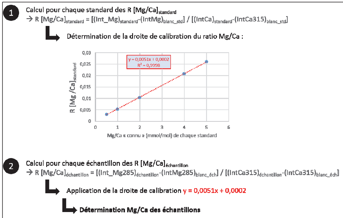
Figure 32 : Illustration de la méthode de calibration dite des ratios d'intensité.
