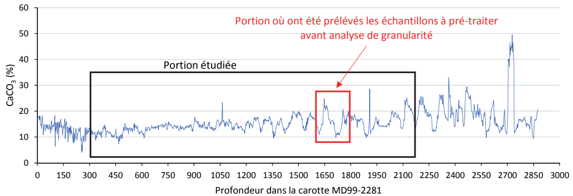
Figure 27 : Evolution du taux de CaCO_3 d'après calibration XRF dans la carotte MD99-2281
