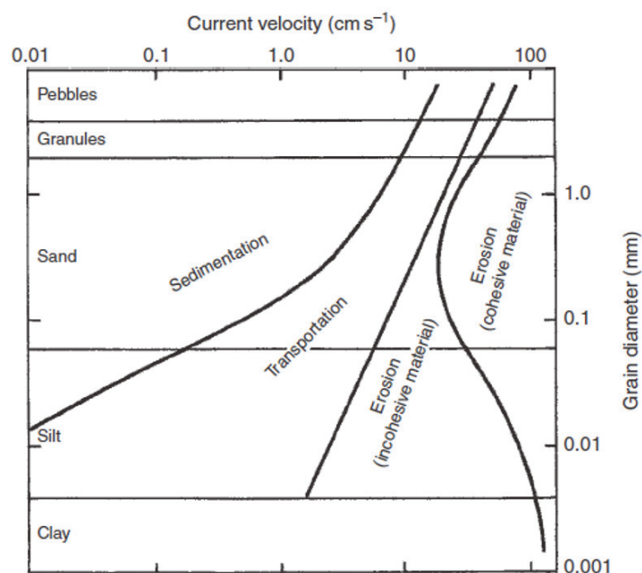
Figure 11 : Représentation simplifiée des vitesses de courant de fond nécessaires pour éroder, transporter et déposer des particules sédimentaires de différentes tailles et différentes natures (issue de Zenk, 2008).
