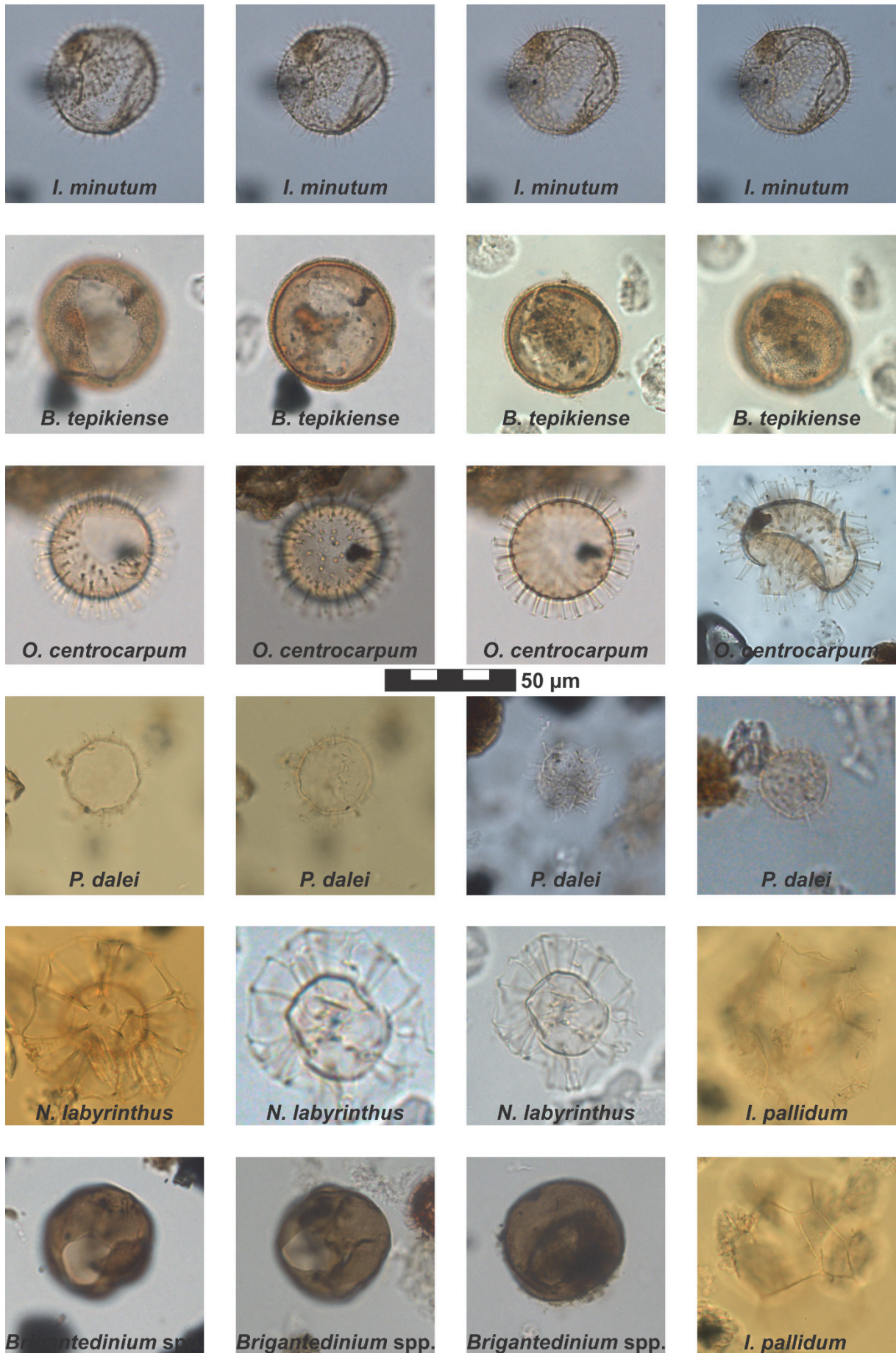
Planche 1 : Micro-photographies de certains taxons de dinokystes rencontrés dans cette thèse.
