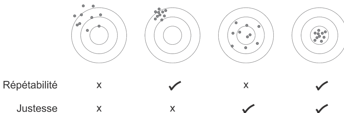
Figure 30 : Notions de justesse et de répétabilité
