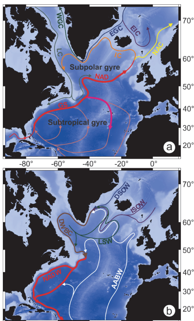
Figure 6 : Circulation océanique en Atlantique Nord. (a) Circulation de surface (GS : Gulf Stream, NAD : North Atlantic Drift, NAC : North Atlantic Current, IC : Irminger Current, LC : Labrador Current, EIC : East Icelandic Current, EGC : East Greenland Current, WGC : West Greenland Current). (b) Circulation intermédiaire et profonde (LSW : Labrador Sea Water, ISOW : Iceland-Scotland Overflow Water, DSOW : Denmark Strait Overflow Water, DWBC : Deep Western Boundary Current, NADW : North Atlantic Deep Water, AABW : Antarctic Bottom Water). Circulation d'après Stanford et al., 2011. Bathymétrie GEBCO ( www.gebco.net ). WGS 1984 Mercator 55°N.
