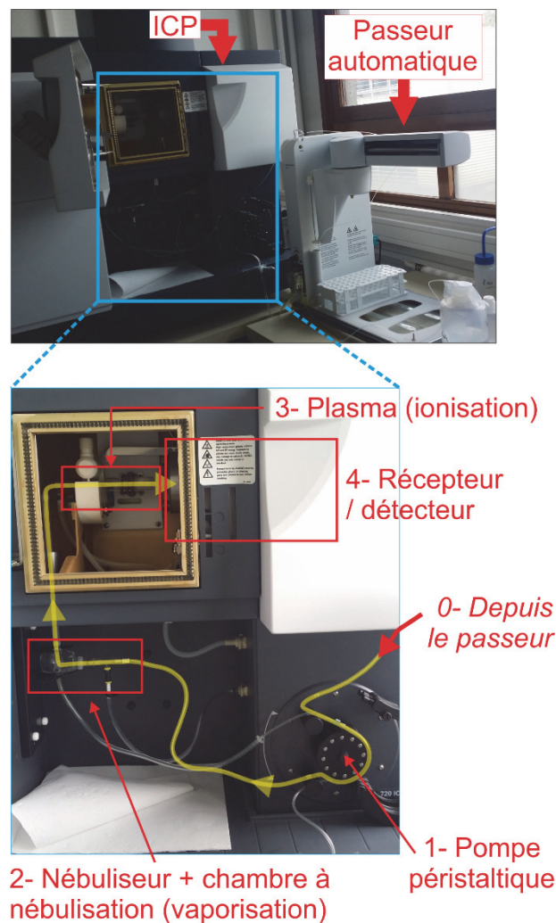
Figure 29 : Schéma de fonctionnement d'un ICP-OES
