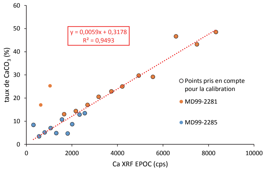
Figure 26 : Résultat des mesures de calcimétrie et droite de calibration Ca (XRF NIOZ) – taux de CaCO_3
