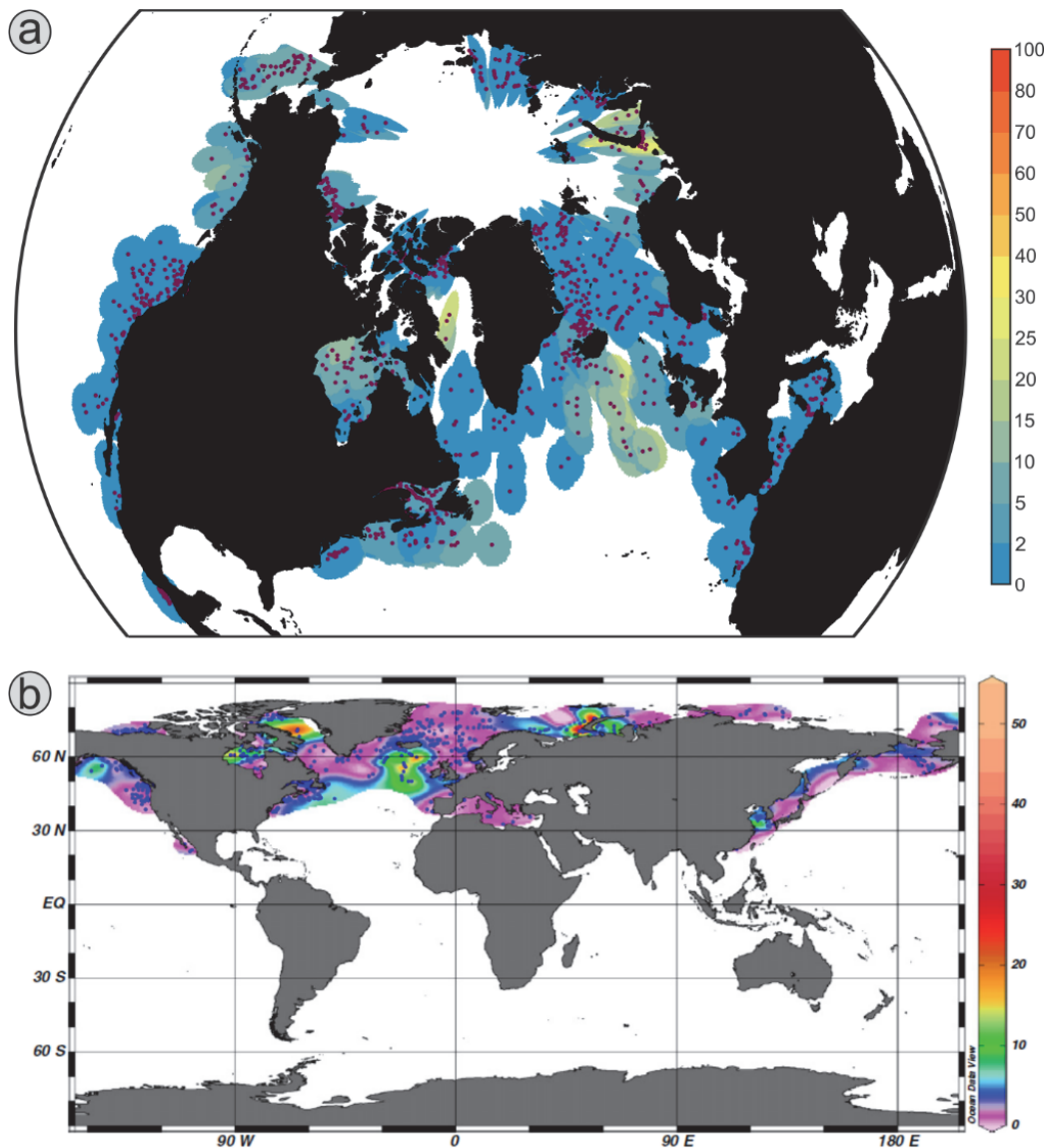
Figure 21 : Cartes de distribution (en pourcentages) de Spiniferites elongatus/S. frigidus (a) dans la base de données modernes n = 1207 , carte construite sous ARCGIS et (b) issue de l'atlas mondial de Zonneveld et al. (2013).
