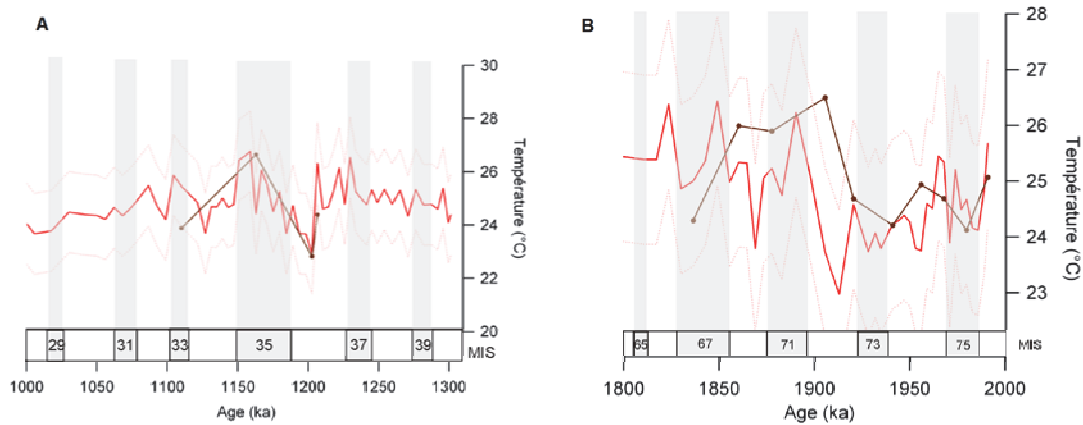
Figure 33 : Comparaison des signaux de température issus de la méthode Mg/Ca sur PF (courbes noires) et de la méthode fonction de transfert sur assemblages de PF (courbes rouges) sur les portions (a) 1 – 1.3 Ma BP et (b) 1.8 – 2 Ma BP de la carotte MD96-2048 (figure modifiée d’après Extier, 2015).
