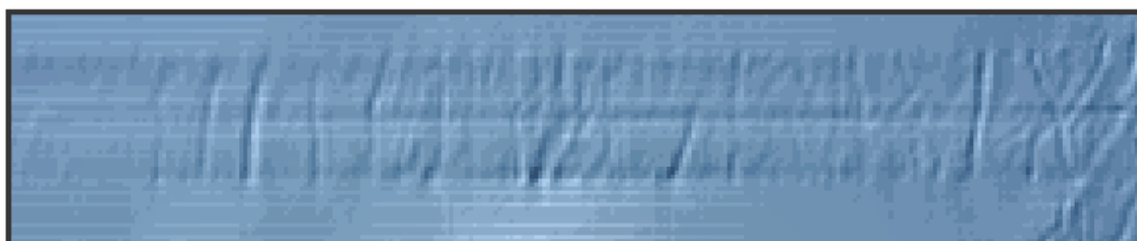
Figure 9 : Iceberg ploughmarks proches de la zone d'étude (localisation indiquée sur la Figure 8b). Données EMODNET ( www.emodnet.eu ).
