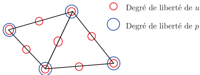
Figure 3 – Représentation des éléments finis de Taylor-Hood en 2D.
