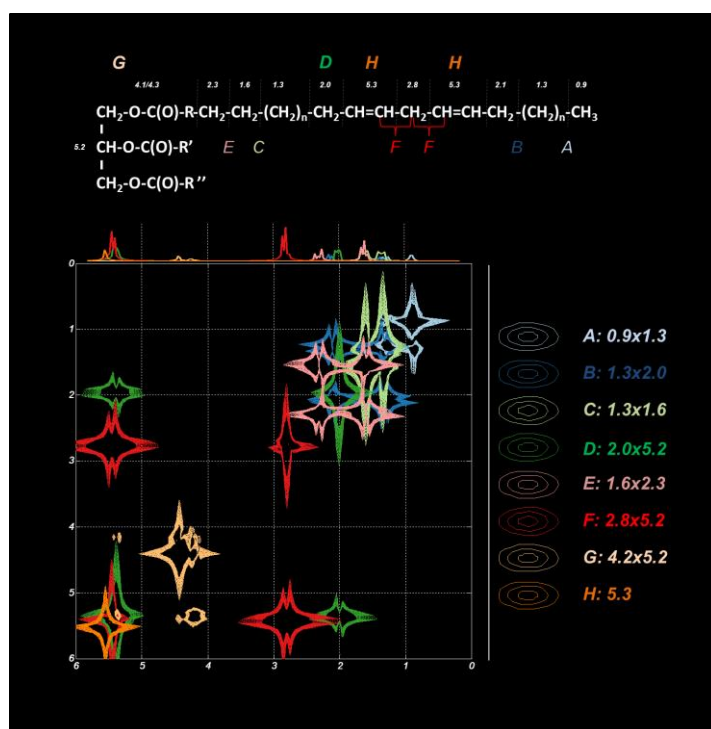
Figure 61 : Base de triglycérides simulée en LCOSY. Les simulations ont été apodisé et normalisés à la même intensité. Les résonances d'un même groupement ont la même couleur de contours.
