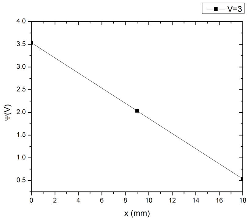
Figure 28: Potentiel électrique pour une polarisation directe de 3 Volts.
