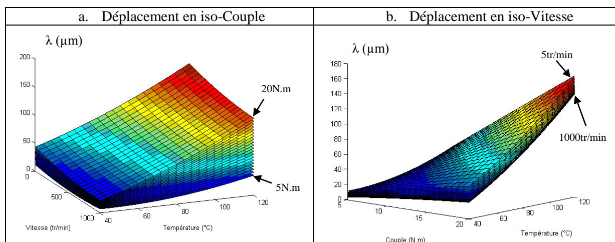
Figure 4.132 : Evolution du déplacement total en tête \lambda
