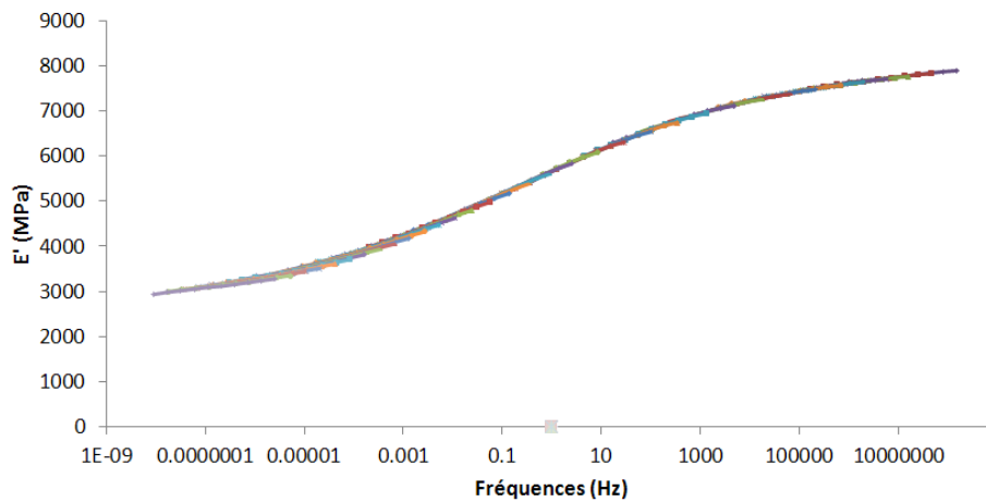
Figure 2.76 : Courbe maîtresse du module de conservation déduite des mesures isothermes de spectrométrie mécanique à une température de référence de 60^{\circ}\text{C} et à sec
