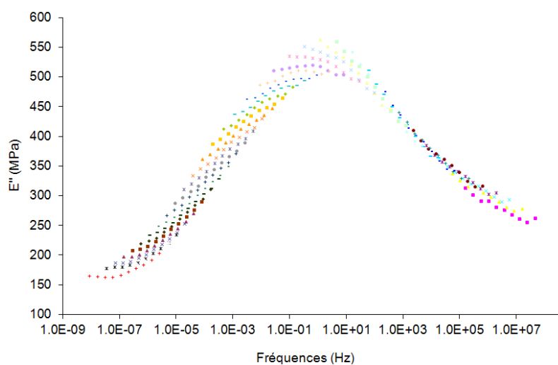
Figure 2.77 : Courbe maîtresse du module de perte déduite des mesures isothermes de spectrométrie mécanique à une température de référence de 60^{\circ}\text{C} et à sec
