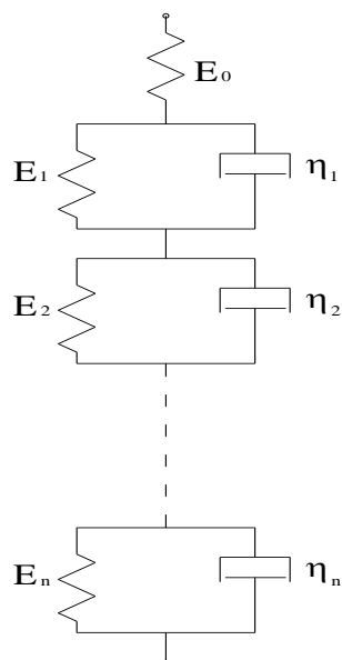
Figure 1.23: Modèle de Kelvin généralisé [10]
