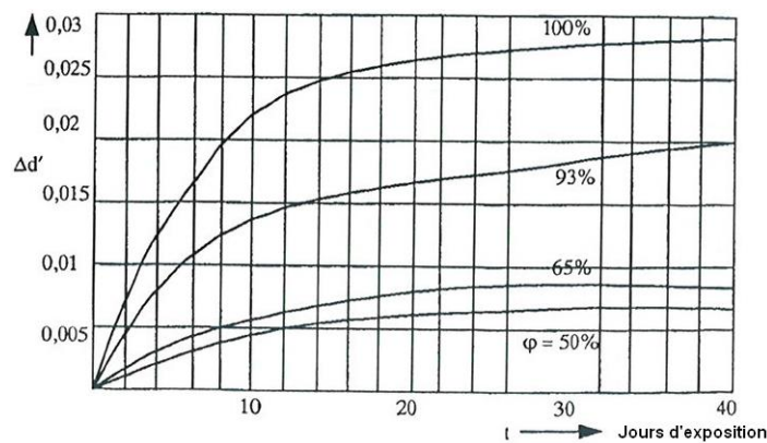
Figure 1.30 : Choix du coefficient \Delta d' en fonction de l'humidité ambiante \varphi et du nombre de jours d'exposition [59]
