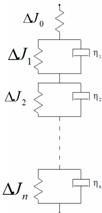
Figure 2.65 : Modèle de Kelvin généralisé
