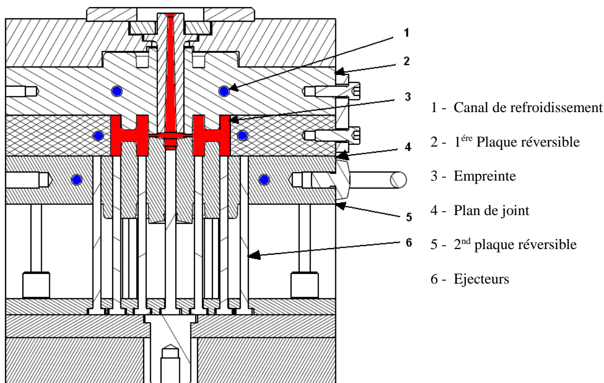
Figure 2.49 : Structure du moule
