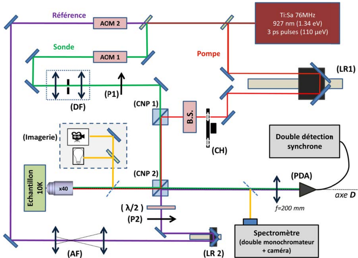
FIGURE 5.2 – Le faisceau laser est divisé en trois faisceaux. Le faisceau pompe (en rouge) est réfléchi sur une ligne à retard (LR1), passe à travers un chopper (CH), et un compensateur Babinet-Soleil (BS), avant d'être réfléchi sur le premier cube non polarisant (CNP1) et puis le deuxième (CNP2), et de rentrer dans l'objectif. Le faisceau sonde (en vert), traverse un modulateur acousto-optique (AOM1), puis un dispositif de filtrage (DF), et un polariseur (P1). Il traverse ensuite CNP1 et est réfléchi sur CNP2, afin de rentrer dans l'objectif superposé spatialement avec la pompe. Sa réflexion à travers l'objectif définit un axe D. Enfin le faisceau référence (en violet) traverse un (AOM2), puis un agrandisseur de faisceau (AF), avant d'être réfléchi sur une petite ligne à retard (LR2). Puis il traverse un polariseur (P2) et une lame ( \lambda/2 ) avant d'être réfléchi sur (CNP2). Cette réflexion est superposée avec l'axe D de réflexion de la sonde, ce qui permet aux deux faisceaux d'interférer sur la photo-diode à avalanche (PDA), sur laquelle ils sont focalisés par une lentille de focale f = 200 mm. La PDA est reliée à la détection synchrone qui permet l'acquisition du signal. On représente aussi sur ce schéma le placement des système d'imagerie et de collection de la photoluminescence de l'expérience (en jaune).
