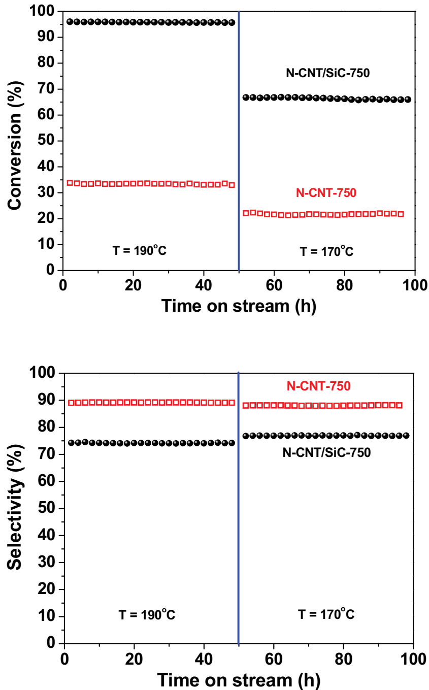
Fig. 3. L'activité en désulfuration de l' \text{H}_2\text{S} en fonction de la température sur des catalyseurs à base de N-NTC/SiC et N-NTCs. Conditions expérimentales: \text{H}_2\text{S} = 1 vol.%; ratio \text{O}_2/\text{H}_2\text{S} = 2,5 ; \text{H}_2\text{O} = 30 vol.%; \text{WHSV} = 0,6 \text{ h}^{-1} ; M_{\text{cata}} (phase active) = 300 mg.
