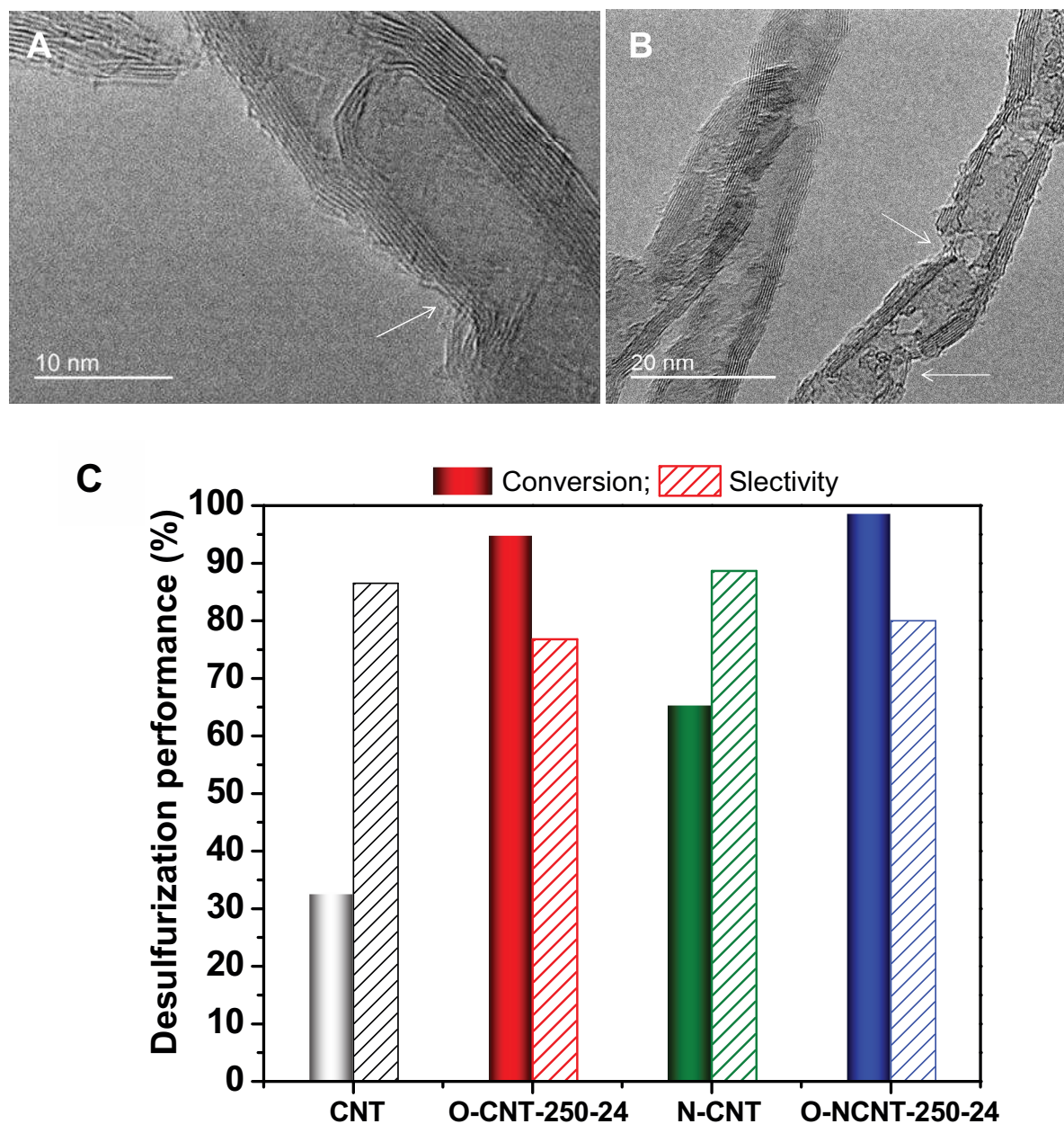
Fig. 5. (A, B) Images MET des nanotubes de carbone présentant des défauts structuraux (indiqués par les flèches) de surface après avoir subi un traitement sous flux gazeux d' \text{HNO}_3 à 250 °C pendant 12 et 24 h. (C) Activité désulfurante des catalyseurs sans métaux traités à 250 °C en fonction du temps. L'activité optimale est obtenue avec un catalyseur à base de NTC traités à 250 °C pendant 24 h. Conditions réactionnelles: \text{H}_2\text{S} = 1 vol.%; \text{H}_2\text{O} = 30 vol.% ; \text{O}_2/\text{H}_2\text{S} = 2.5; T = 230 °C; \text{WHSV} = 0.6 \text{h}^{-1} ; M_{\text{cata}} = 300 mg.
