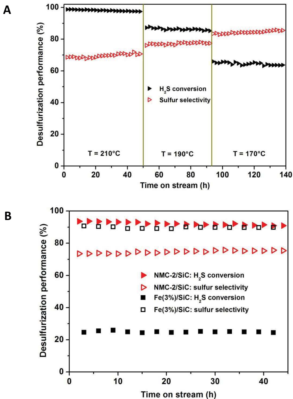
Fig. 4. (A) L'activité en désulfuration de l' \text{H}_2\text{S} obtenue à WHSV de 0.6 \text{ h}^{-1} sur des catalyseurs à base de NMC/SiC en fonction de la température de réaction, et (B) en comparaison avec un catalyseur Fe/SiC. Conditions réactionnelles: T = 210 \text{ }^\circ\text{C} ; WHSV = 0,6 \text{ h}^{-1} , \text{H}_2\text{S} = 1 \text{ vol.}\% ; \text{O}_2/\text{H}_2\text{S} = 2,5 ; \text{H}_2\text{O} = 30 \text{ vol.}\% ; M_{\text{cata}} (phase active) = 300 \text{ mg} .
