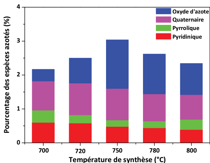
Fig. 2. Diagramme montrant les répartitions des groupements azotés présents dans le N-NTC obtenues par XPS en fonction de la température de synthèse.
