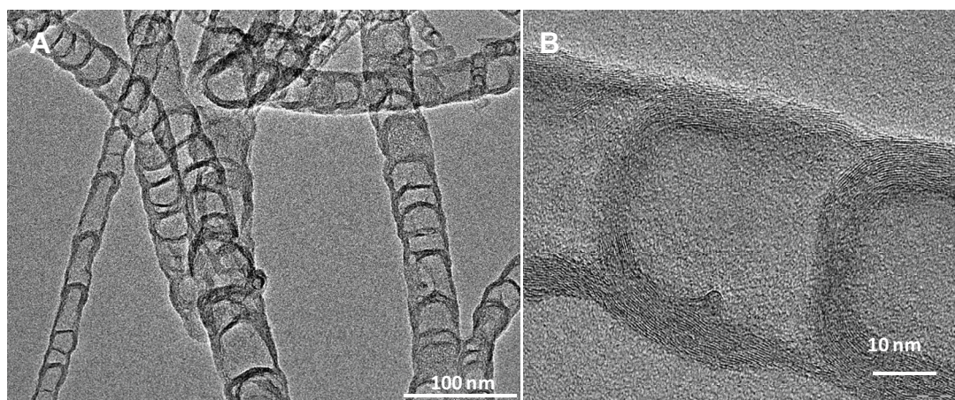
Fig. 1. Images MET des nanotubes de carbone dopés avec de l'azote montrant la morphologie particulière en forme de bambou de ces matériaux et une bonne graphitisation des murs.
